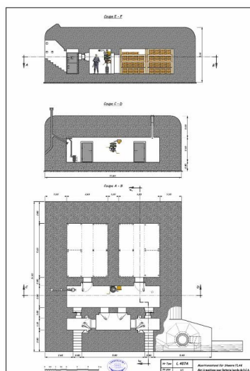
Plan et coupes d'un bunker-abri-magasin de munitions de type L 407a pour batterie antiaérienne (Munitionsstand für 8,8 oder 10,5 cm Flak) Dess. Christian Moigne IVR53_20263510106NUDA
