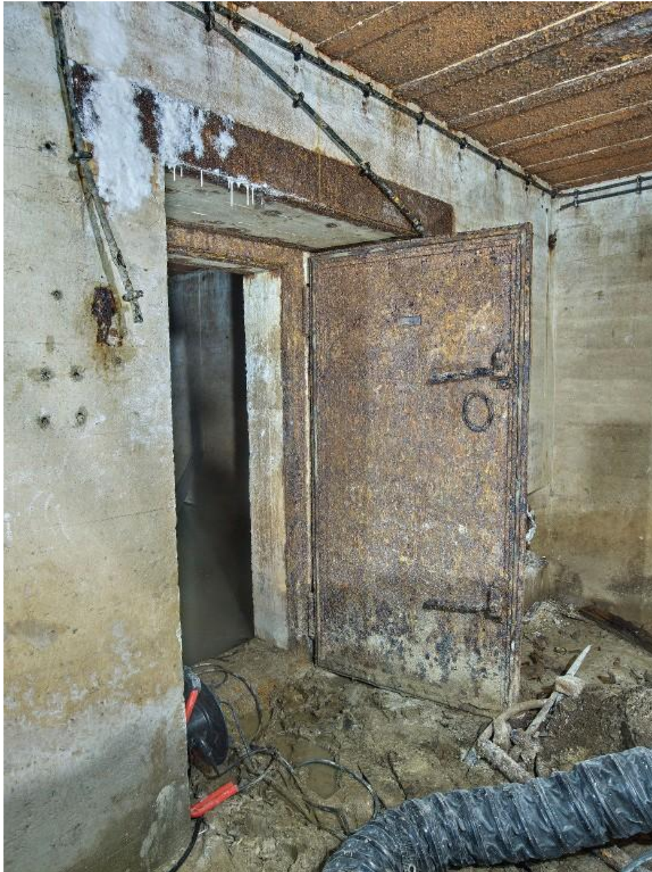
Vue de détail de la porte blindée étanche du magasin à munitions est (cette pièce est partiellement inondée). A gauche, emplacement d'un boîtier électrique : seul le câblage subsiste
