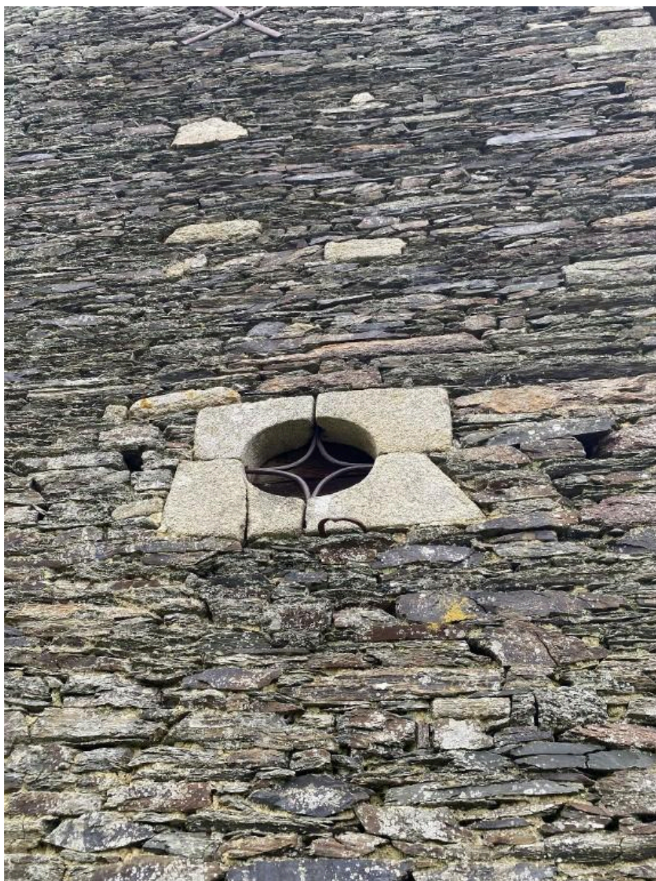
Oculus, pignon sud, détail
