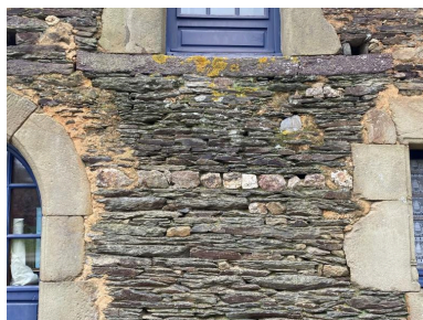
Aile nord, détail Phot. Baptiste Oligo IVR53_20265610199NUCA
