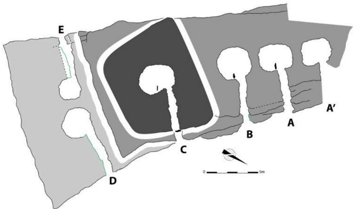
île Guénioec : Évolution du cairn III de Guénioec au fil du temps, du plus foncé au plus clair
