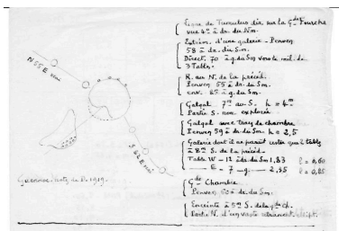
île Guénioec : Premier relevé archéologique sur l'île Guennoc par E. Morel Phot. Auteur inconnu (phototype/graphique) IVR53_20242911544NUCA
