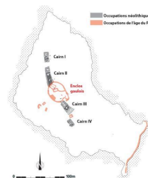
île Guénioec : Plan de répartition des vestiges présents sur l'île Guénioec Phot. Florian Cousseau IVR53_20242911543NUCA
