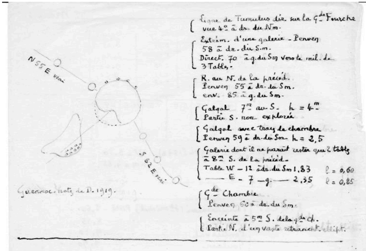
île Guénioec : Premier relevé archéologique sur l'île Guennoc par E. Morel
