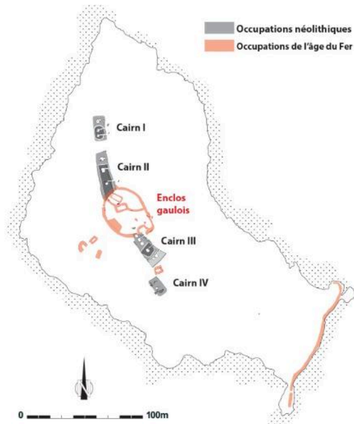
île Guénioec : Plan de répartition des vestiges présents sur l'île Guénioec
