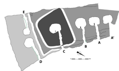
île Guénioec : Évolution du cairn III de Guénioec au fil du temps, du plus foncé au plus clair Phot. Florian Cousseau IVR53_20242911540NUCA
