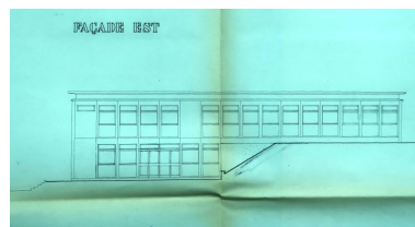
IVR53_20193505600A0 Infirmerie, élévation de la façade est, J. Monge et R. Guichebaron, architectes, 1964. Dess. Jean Monge, Dess. René Guichebaron, Autr. Thierry Goyet IVR53_20193505605A0
