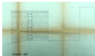
Élévation du pignon est d'un externat (ici bâtiment H), Monge [J.], Guichebaron [R.], architectes, 1964. Dess. Jean Monge, Dess. René Guichebaron, Autr. Thierry Goyet
