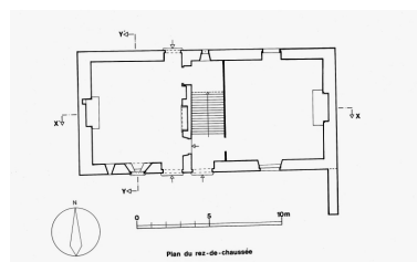
Plan du rez-de-chaussée. Phot. Guy Artur, Phot. Norbert Lambart IVR53_19863500051P
