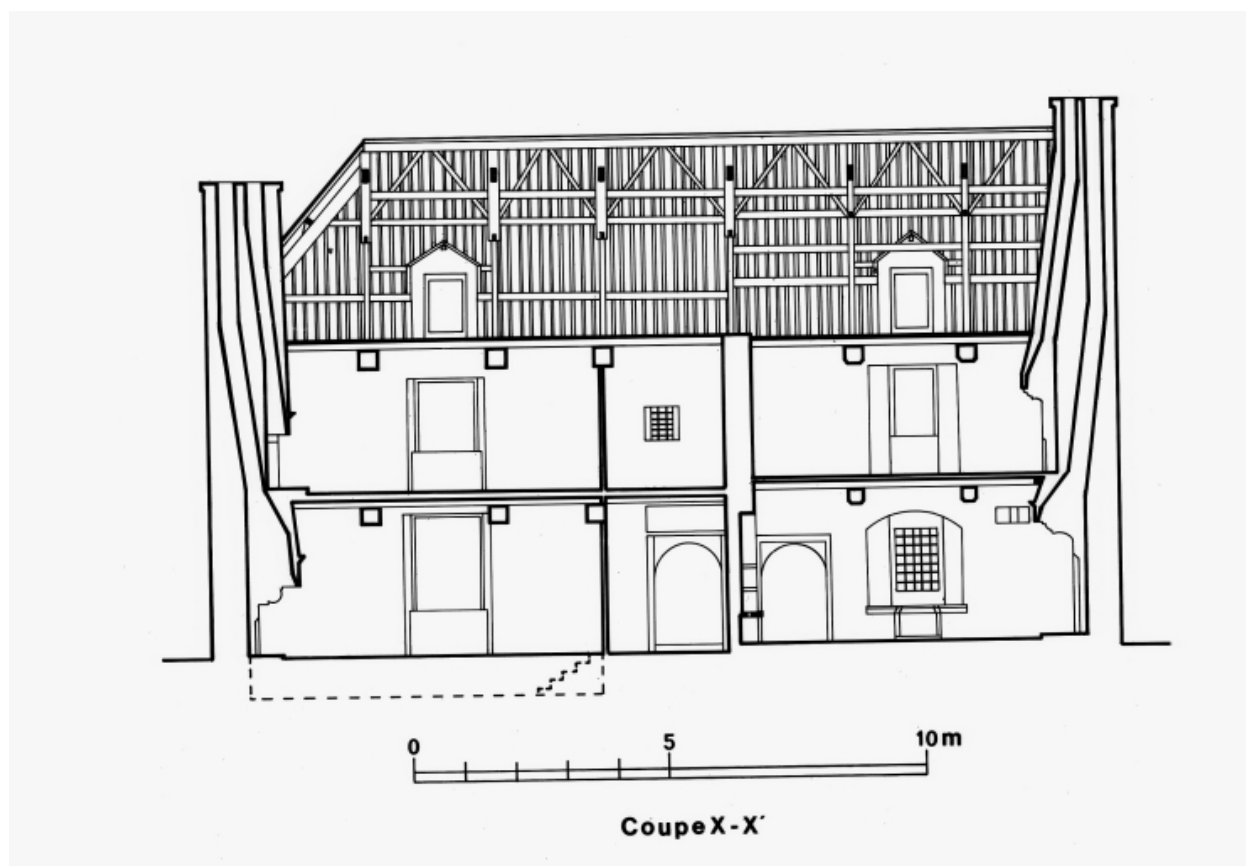
Coupe XX'.
