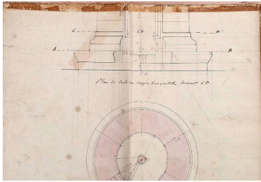
Plan du socle du phare de la pointe de l'Aigle (18 novembre 1855) Repro. Erwana L'Haridon IVR53_20262210097NUCA
