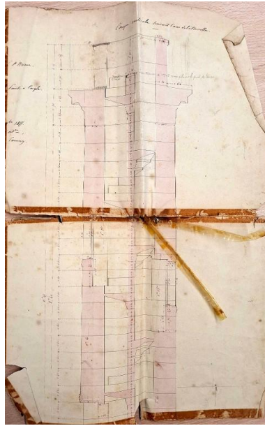
Coupe verticale du phare de la pointe de l'Aigle (18 novembre 1855) Repro. Erwana L'Haridon IVR53_20262210095NUCA
