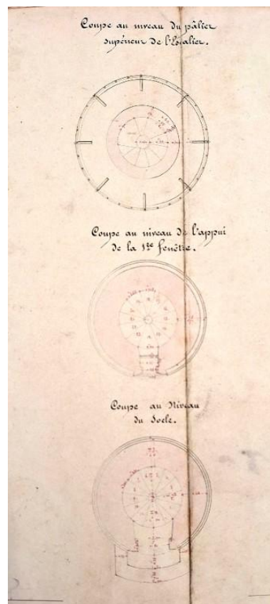
Coupe du phare de la pointe de l'Aigle de chaque niveau (29 novembre 1851) Repro. Erwana L'Haridon, Autr. Gayffrier, Autr. Camus IVR53_20262210108NUCA
