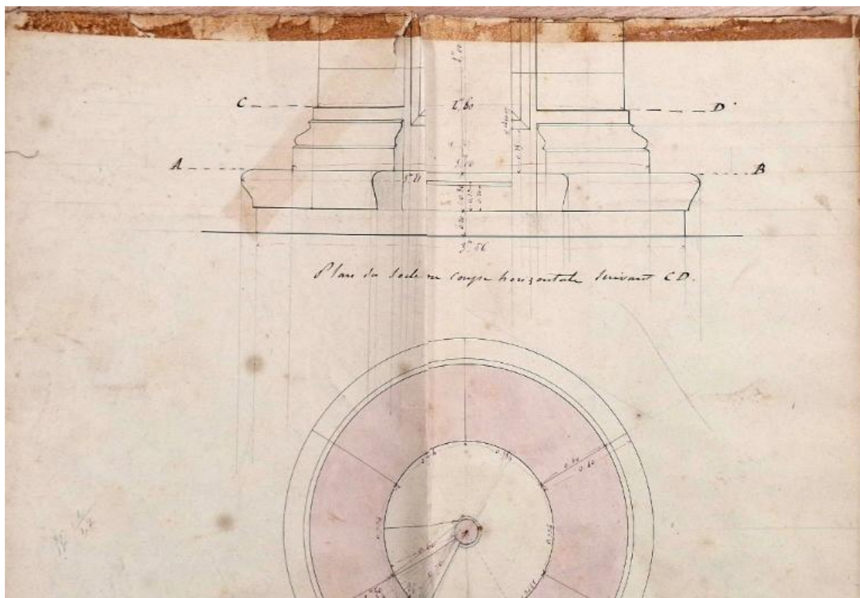
Plan du socle du phare de la pointe de l'Aigle (18 novembre 1855)
