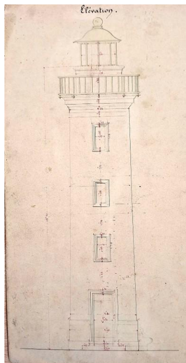
Elévation du phare de la pointe de l'Aigle (29 novembre 1851) Repro. Erwana L'Haridon, Autr. Gayffrier, Autr. Camus IVR53_20262210102NUCA
