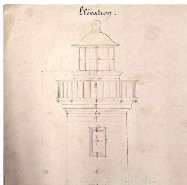
Plan : élévation du phare de la pointe de l'Aigle, 29 novembre 1851 (extrait) Repro. Erwana L'Haridon, Autr. Gayffrier, Autr. Camus IVR53_20262210110NUCA
