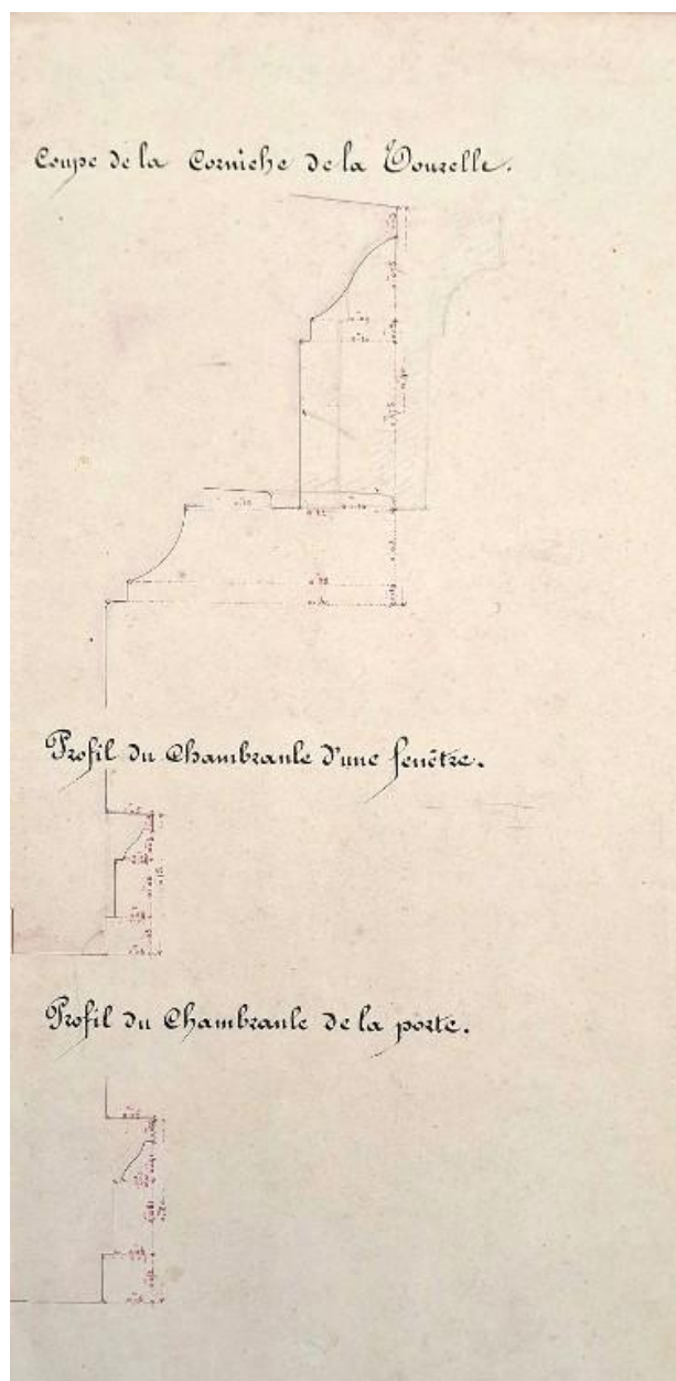
Profils des corniches et chambranles du phare de la pointe de l'Aigle (29 novembre 1851)
