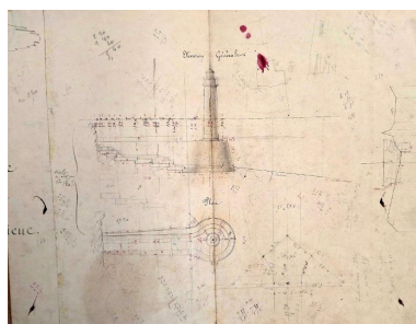
Elévation générale du phare de la pointe de l'Aigle (1851) Repro. Erwana L'Haridon, Autr. Gayffrier, Autr. Camus IVR53_20262210104NUCA
