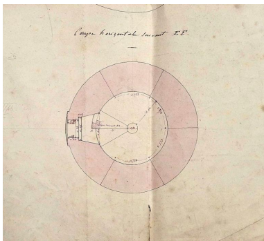
Coupe horizontale du phare de la pointe de l'Aigle (18 novembre 1855) Repro. Erwana L'Haridon IVR53_20262210098NUCA
