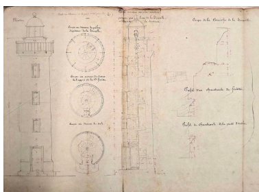
Elévation, coupe et profil du phare de la pointe de l'Aigle (29 novembre 1851) Repro. Erwana L'Haridon, Autr. Gayffrier, Autr. Camus IVR53_20262210105NUCA
