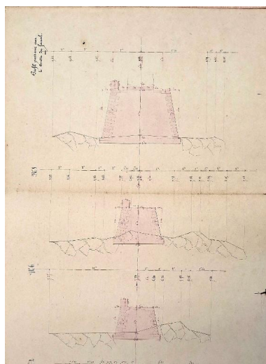
Profil de la jetée du phare de la pointe de l'Aigle (29 novembre 1851) Repro. Erwana L'Haridon, Autr. Gayffrier, Autr. Camus IVR53_20262210099NUCA
