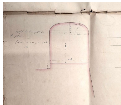
Profil du parapet de la jetée du phare de la pointe de l'Aigle (7 novembre 1855) Repro. Erwana L'Haridon IVR53_20262210107NUCA
