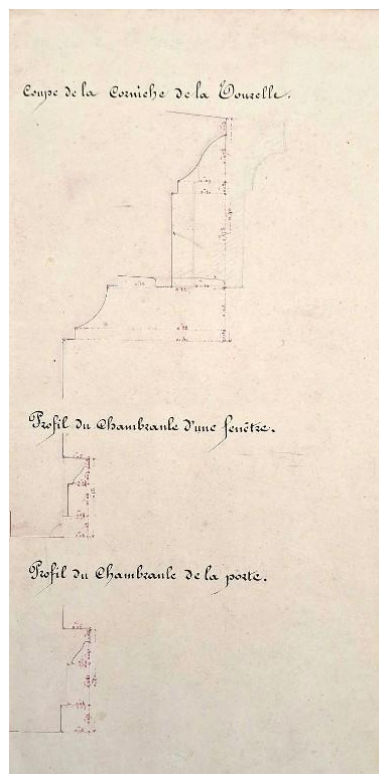
Profil des corniches et chambranles du phare de la pointe de l'Aigle (29 novembre 1851) Repro. Erwana L'Haridon, Autr. Gayffrier, Autr. Camus IVR53_20262210103NUCA
