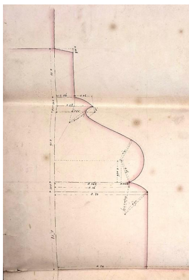
Profil des corniches du phare de la pointe de l'Aigle (18 novembre 1855) Repro. Erwana L'Haridon IVR53_20262210101NUCA
