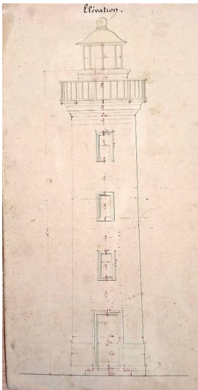
Elévation du phare de la pointe de l'Aigle (29 novembre 1851)
