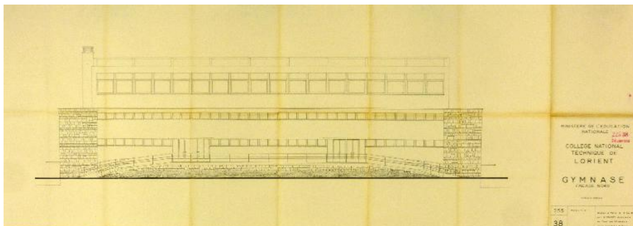
Façade nord
