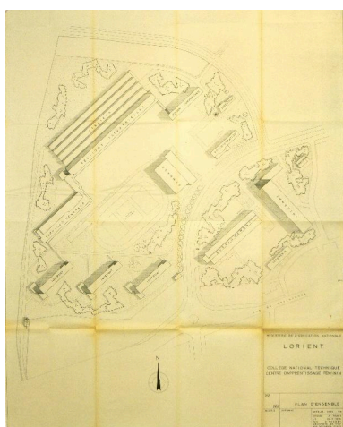
Plan d'ensemble du collège national technique Phot. Philippe Bonnet IVR53_20185605035NUCA
