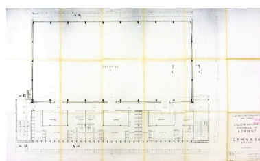
Plan du gymnase (étage) Phot. Philippe Bonnet IVR53_20185605037NUCA
