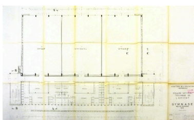
Plan du gymnase (rez- de-chaussée bas) Phot. Philippe Bonnet IVR53_20185605036NUCA
