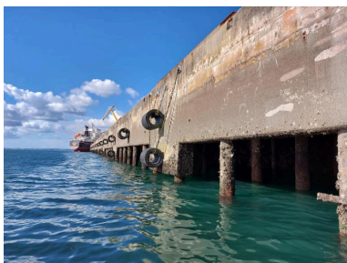
Quai sur pieux de la plate-forme multimodale Phot. Région Bretagne IVR53_20222906321NUCA
