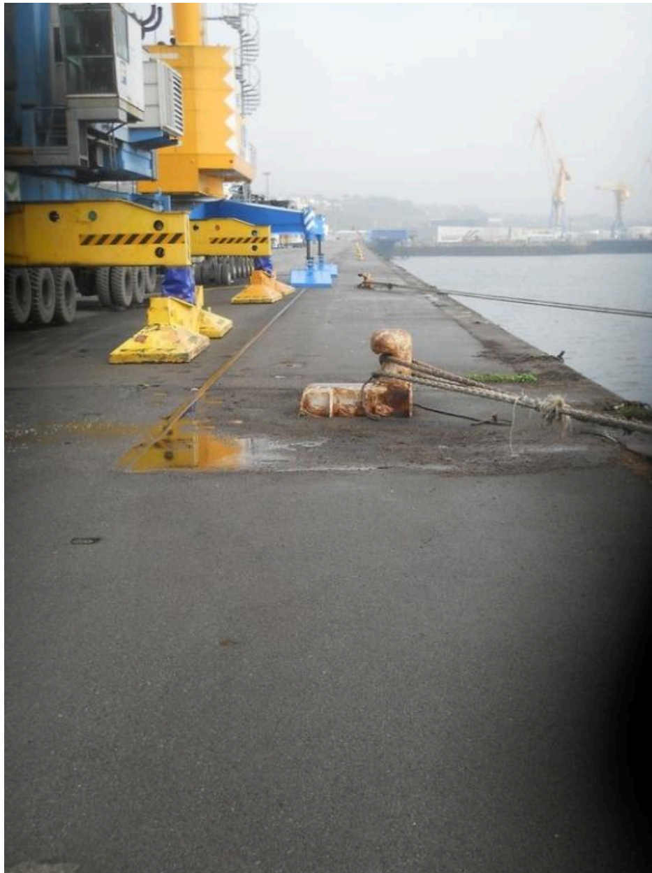
Plate-forme multimodale, grues Reggiane, appuis, bollards
