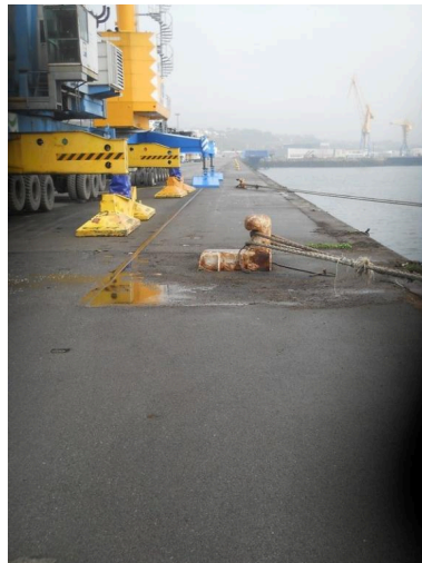
Plate-forme multimodale, grues Reggiane, appuis, bollards Phot. Région Bretagne IVR53_20222906320NUCA
