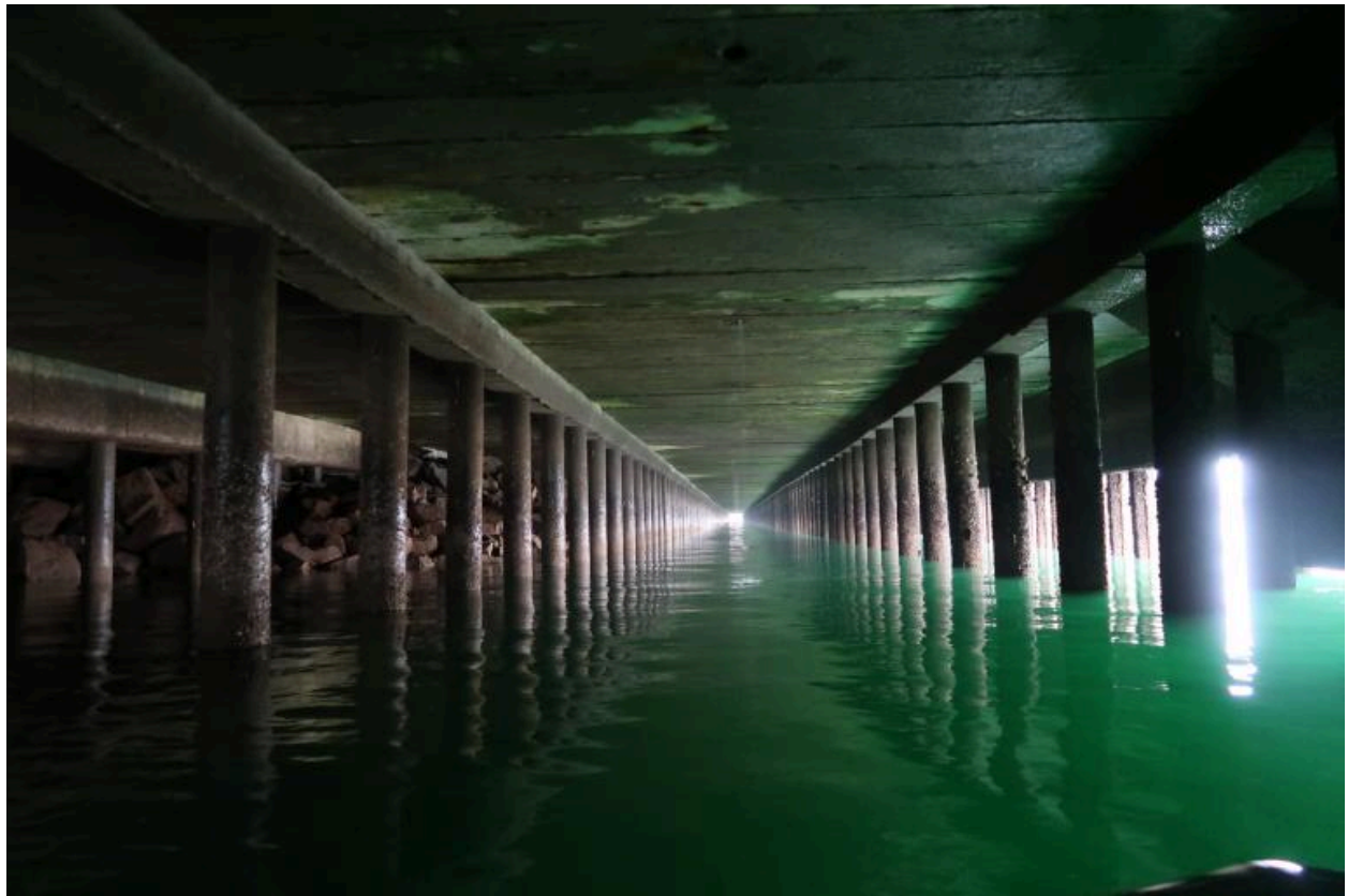
Passage sous la plate-forme multimodale : dalles, pieux.
