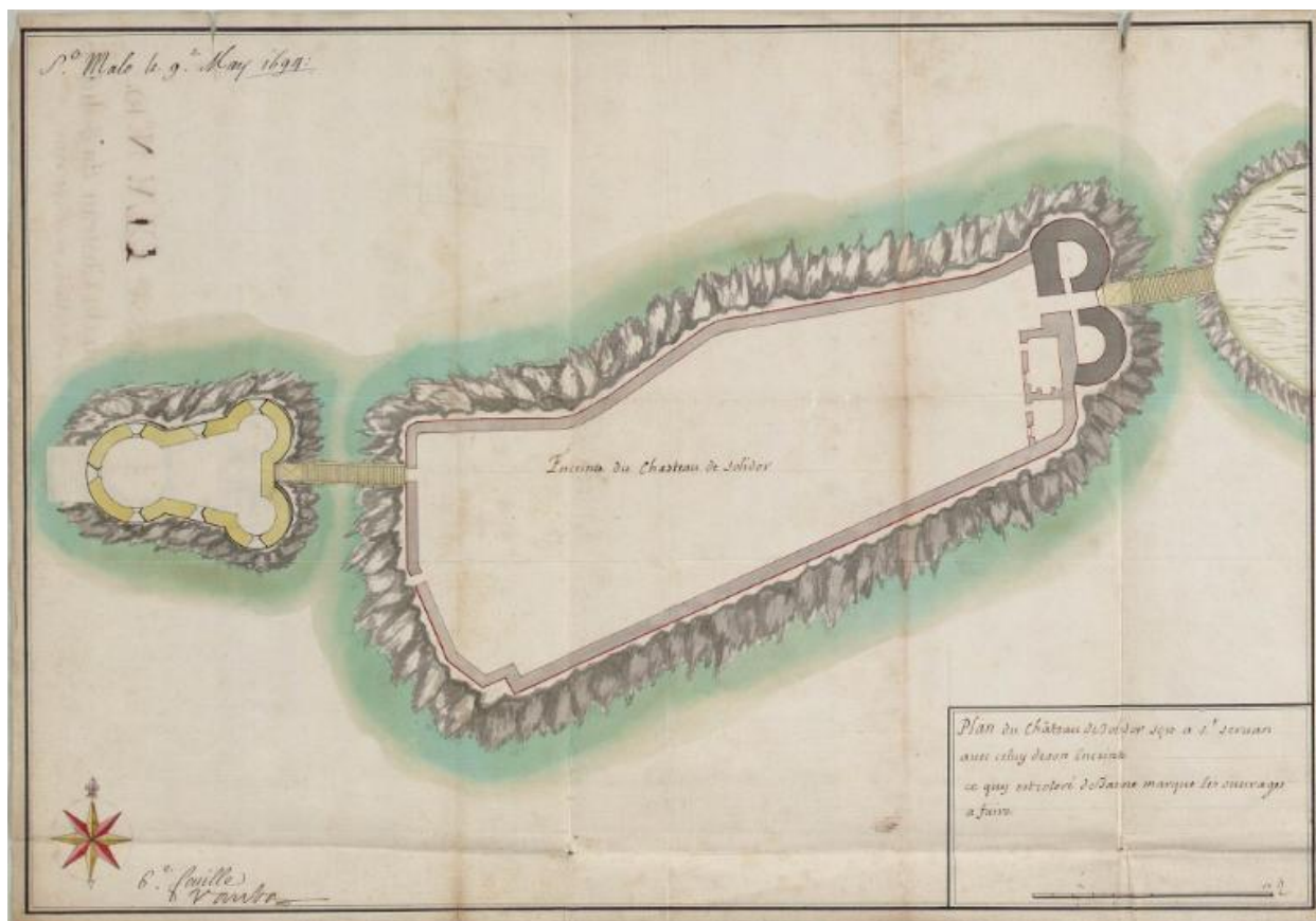
Plan de la plate-forme d'artillerie de la Tour Solidor et de son ouvrage avancé contresigné par Vauban, 9 mai 1694. Lavé de jaune, le projet
