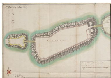
Plan de la plate-forme d'artillerie de la Tour Solidor et de son ouvrage avancé contresigné par Vauban, 9 mai 1694. Lavé de jaune, le projet Repro. Auteur inconnu, Autr. Sébastien Le Prestre de Vauban, Autr. Siméon Garengneau IVR53_20253510292NUCA
