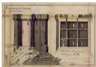
Elévation et coupe de la Tour Solidor par l'ingénieur Garengneau, 27 janvier 1697. Lavé de jaune, le projet Repro. Auteur inconnu, Autr. Siméon Garengneau IVR53_20253510297NUCA
