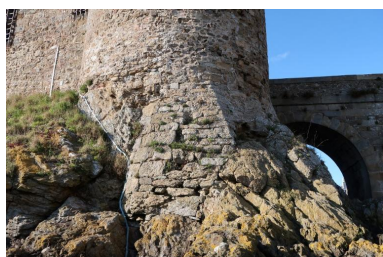
Vue du pied de la tour est : la maçonnerie est très dégradée. A droite, le pont dormant Phot. Guillaume Lécueillier IVR53_20263510556NUCA
