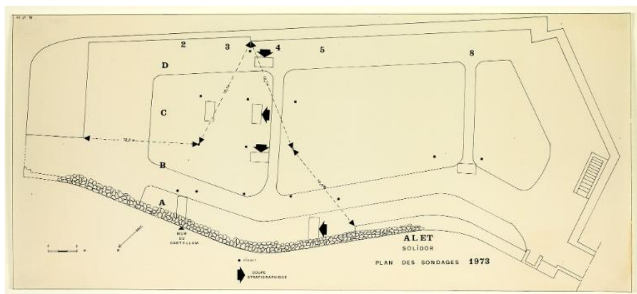
Plan des sondages archéologiques sur l'ouvrage avancé de la Tour Solidor, 1973
