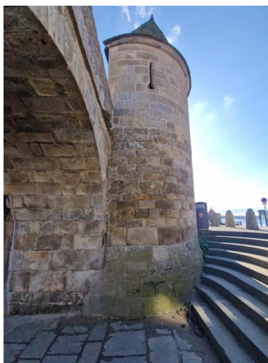
Vue de la tour nord du châtelet d'entrée de la basse-cour. La partie haute de la tour a fortement été restaurée. A gauche, le pont dormant de la basse-cour Phot. Guillaume Lécueillier IVR53_20263510531NUCA
