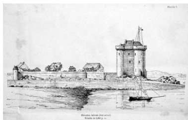
Vue de la tour Solidor depuis le nord-ouest : état avant restauration, dessin d'Albert Ballu, architecte, planche n° 7, 1883. Au sommet de tour se dresse un mât de pavillon. Dans la basse-cour se trouvent deux bâtiments. Les arches du pont sont occupées Phot. Auteur inconnu (phototype/graphique) IVR53_20253510325NUC
