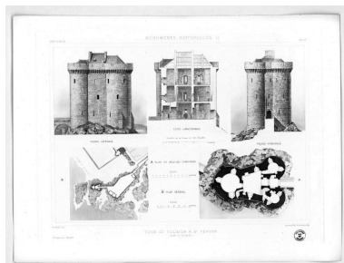
Monuments historiques II. 14e siècle. Planche 53. Tour de Solidor à Saint-Servan (Ile-et-Vilaine). Façade latérale. Coupe longitudinale. Façade principale. Plan du rez-de-chaussée. Plan général. (Albert Ballu ; héliogravure Chauvet)
