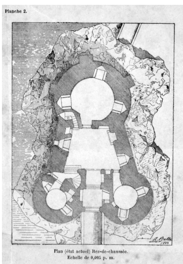
Plan du rez-de-chaussée de la tour Solidor : état avant restauration, dessin d'Albert Ballu, architecte, planche n° 2, 1883 Phot. Auteur inconnu (phototype/graphique) IVR53_20253510320NUC
