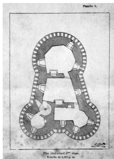
Plan du 2e étage de la tour Solidor : état avant restauration, dessin d'Albert Ballu, architecte, planche n° 3, 1883 Phot. Auteur inconnu (phototype/graphique) IVR53_20253510321NUC
