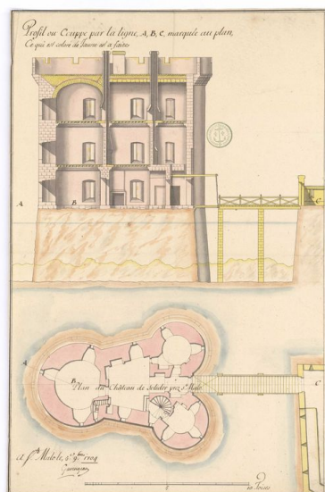
Plan, profil et coupe de la Tour Solidor, fait à Saint-Malo le 5 novembre 1704 par Garangeau Repro. Service historique de la Défense, Autr. Siméon (Simon) Garengneau IVR53_20083510498NUCA
