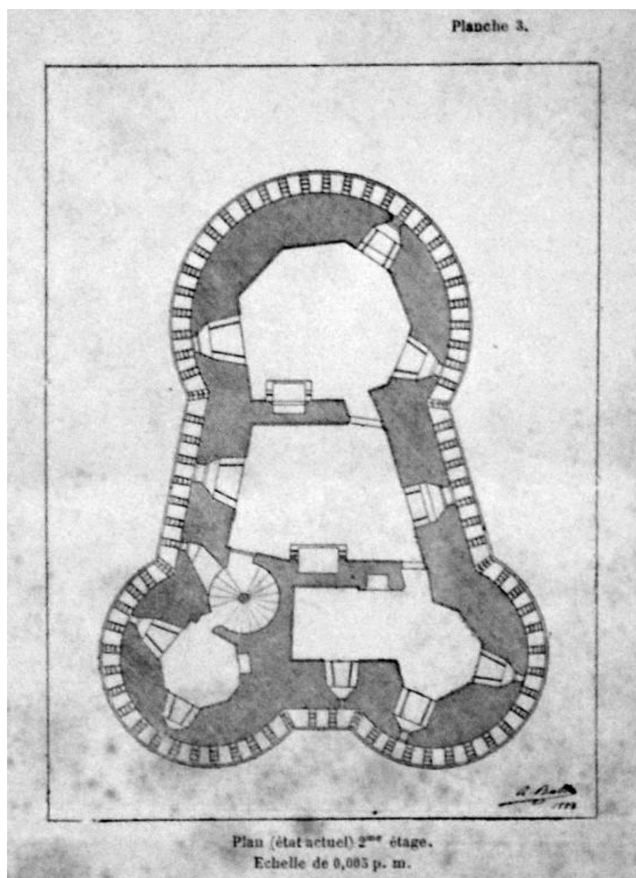
Plan du 2e étage de la tour Solidor : état avant restauration, dessin d'Albert Ballu, architecte, planche n° 3, 1883
