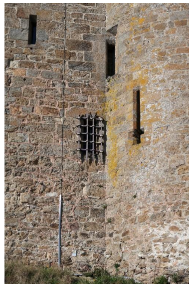
Vue de détail de l'élévation sud de la tour. Au rez-de-chaussée : jour grillée de la cage d'escalier et arbalétrière-canonnière de la tour est (dépourvue d'arc de décharge). En haut, jours/arbalétrières de la cage d'escalier au niveau intermédiaire Phot. Guillaume Lécueillier IVR53_20263510553NUCA
