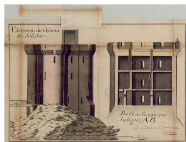
Elévation et coupe de la Tour Solidor par l'ingénieur Garengneau, 27 janvier 1697. Lavé de jaune, le projet Repro. Auteur inconnu, Autr. Siméon Garengneau IVR53_20253510298NUCA
