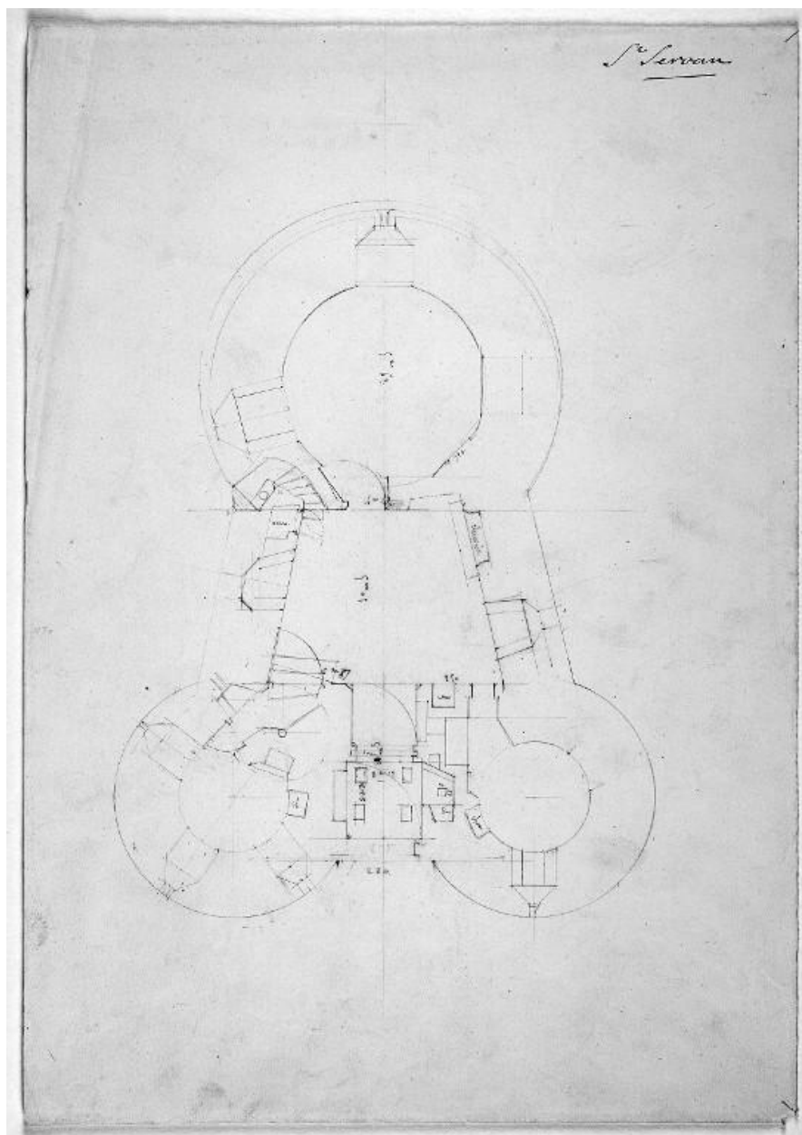
Plan du rez-de-chaussée de la Tour Solidor par Alfred Ramé
