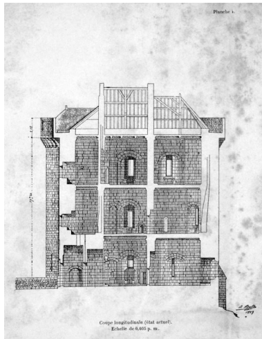
Coupe longitudinale de la tour Solidor : état avant restauration, dessin d'Albert Ballu, architecte, planche n° 4, 1883 Phot. Auteur inconnu (phototype/graphique) IVR53_20253510322NUC
