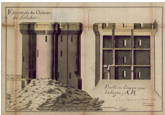
Elévation et coupe de la Tour Solidor par l'ingénieur Gareneau, 27 janvier 1697. Lavé de jaune, le projet
