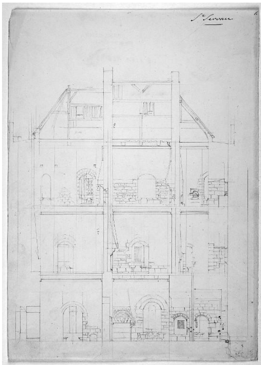
Coupe longitudinale de la Tour Solidor par Alfred Ramé
