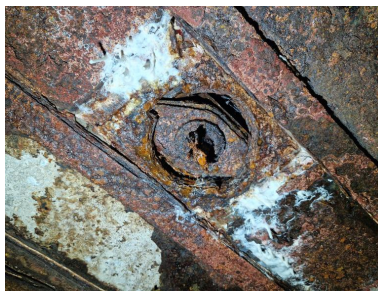
Vue intérieure : petite salle du périscopes, conduit pour le périscopes aménagé dans le plafond. Son système de fermeture est en place Phot. Guillaume Lécueillier IVR53_20242911264NUCA
