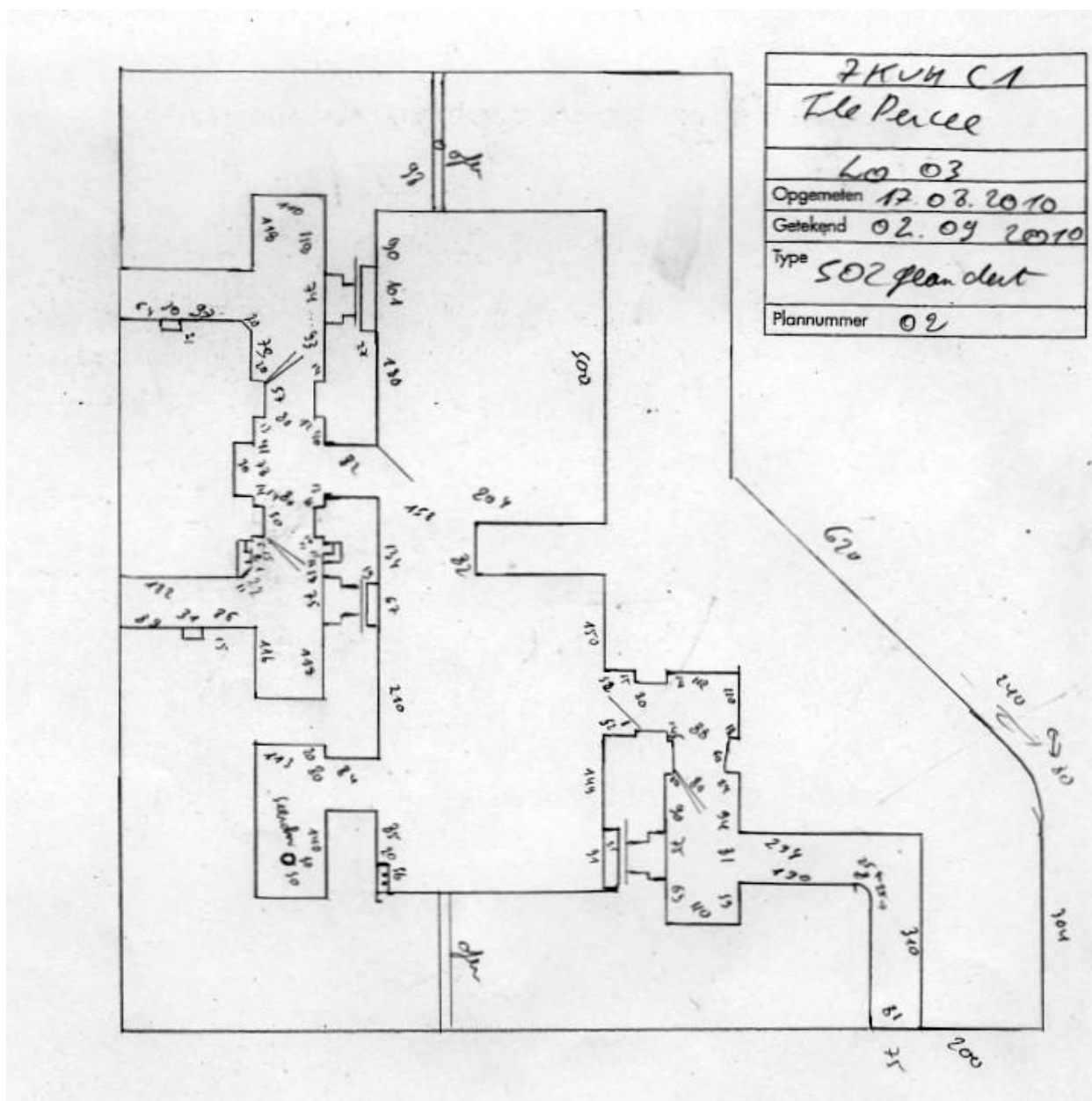
Plan du bunker - abri de type 502 de l'Île Percée (dessin : Dirk Peeters ; collection : Association Mémoire Patrimoine - Clohars-Carnoët)
