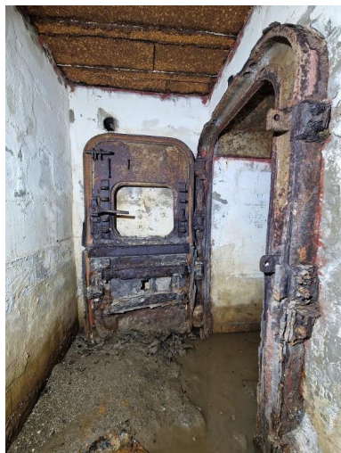
Vue intérieure : petite salle du périscopes, porte blindée à deux vantaux Phot. Guillaume Lécueillier IVR53_20242911263NUCA
