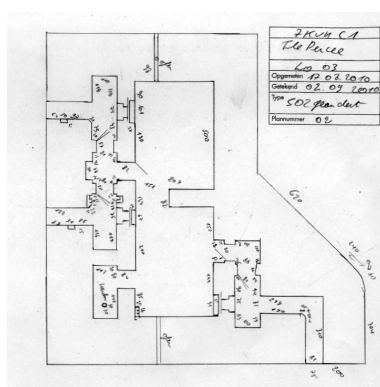
Plan du bunker - abri de type 502 de l'île Percée (dessin : Dirk Peeters ; collection : Association Mémoire Patrimoine - Clohars-Carnoët) Phot. Dirk Peeters IVR53_20242911471NUC
