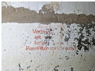
Vue intérieure : salle de garde est, emplacement du ventilateur et marquage en allemand Phot. Guillaume Lécueillier IVR53_20242911266NUCA
