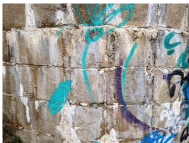
Vue de détail au sud-est. Le bunker est construit avec des parpaings dans lesquels a été coulé le béton. Il est tagué Phot. Guillaume Lécueillier IVR53_20242911228NUCA
