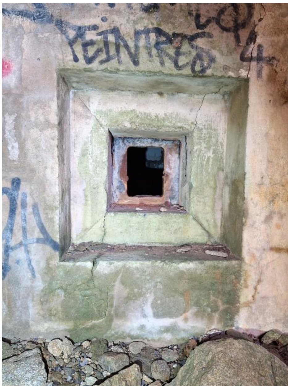
Vue intérieure : accès nord (entrée est) défendue par un créneau blindé
