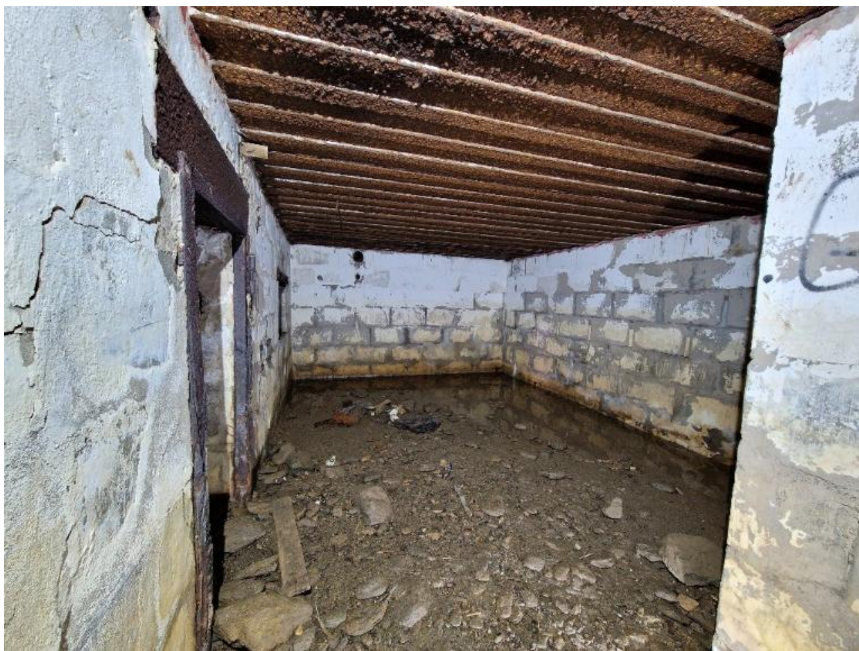
Vue intérieure : salle de garde est. Le bunker est construit avec des parpaings dans lesquels a été coulé le béton
