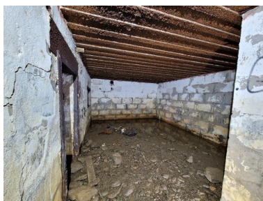
Vue intérieure : salle de garde est. Le bunker est construit avec des parpaings dans lesquels a été coulé le béton Phot. Guillaume Lécueillier IVR53_20242911272NUCA
