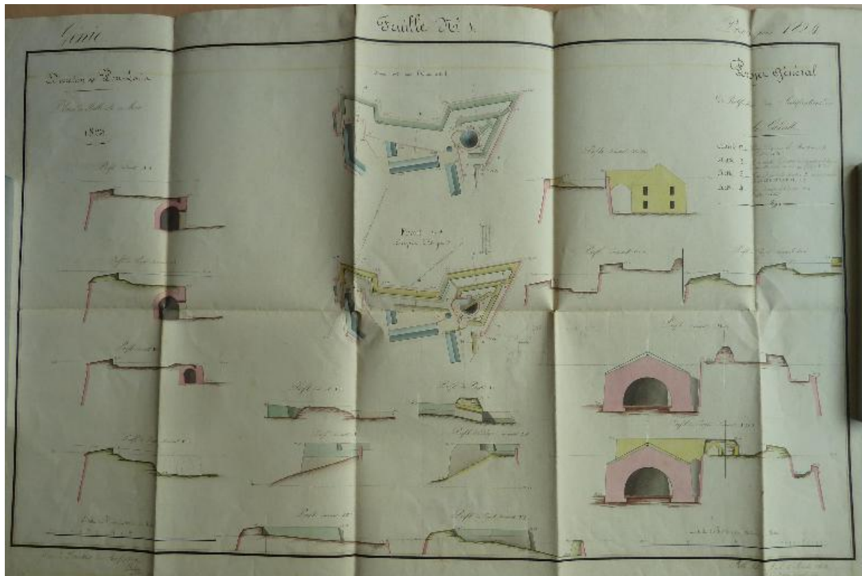
1 VH 287. Place de Belle-Île-en-Mer, feuille n° 1 des projets pour 1824, projet général de rectification des fortifications de la citadelle, 15 novembre 1823.
