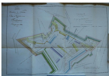
1 VH 289. Place de Belle-Ile-en-Mer, feuille n° 1 des projets pour 1831, plan des travaux à effectuer pour le défilement de la citadelle de Belle-Île-en-Mer, 15 octobre 1830.
