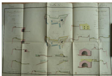
1 VH 287. Place de Belle-Ile-en-Mer, feuille n° 1 des projets pour 1824, projet général de rectification des fortifications de la citadelle, 15 novembre 1823.
