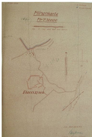
Plan de situation de l'ensemble fortifié n° 92 a près de Créac'h ar Vilin Phot. Guillaume Lécueillier IVR53_20022901977NUCA
