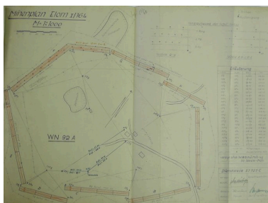
Plan de l'ensemble fortifié n° 92 a près de Créac'h ar Vilin Phot. Guillaume Lécueillier IVR53_20022901978NUCA
