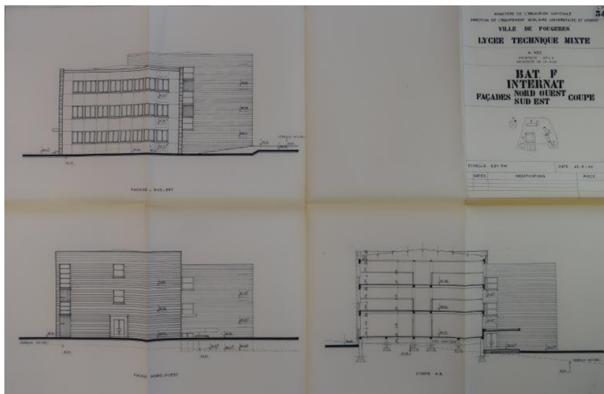
Bâtiment F, Internat. Façades nord-ouest et sud-est et Coupe. Albert Hec, architecte. 1964.
