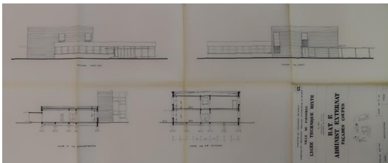
Bâtiment E, Administration - Externat. Façades - Coupes. Albert Hec, architecte. 1964.
