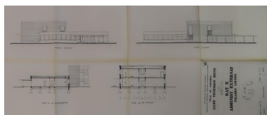
Bâtiment E, Administration - Externat. Façades - Coupes. Albert Hec, architecte. 1964. Autr. Albert Hec IVR53_20203505074A1
