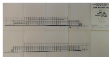
Bâtiment G, Ateliers. Façades nord-est - sud-ouest. Albert Hec, architecte. 1964. Autr. Albert Hec IVR53_20203505079A1
