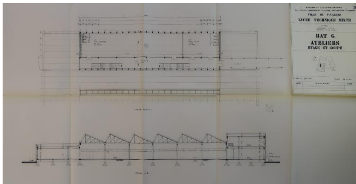
Bâtiment G, Ateliers. Étage et coupe. Albert Hec, architecte. 1964.
