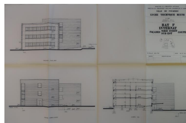
Bâtiment F, Internat. Façades nord-ouest et sud-est et Coupe. Albert Hec, architecte. 1964. Autr. Albert Hec IVR53_20203505076A1
