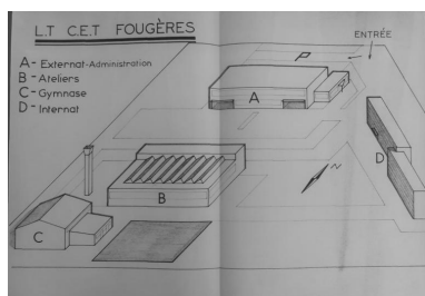
Plan de masse : axonométrie. IVR53_20203505081A3
