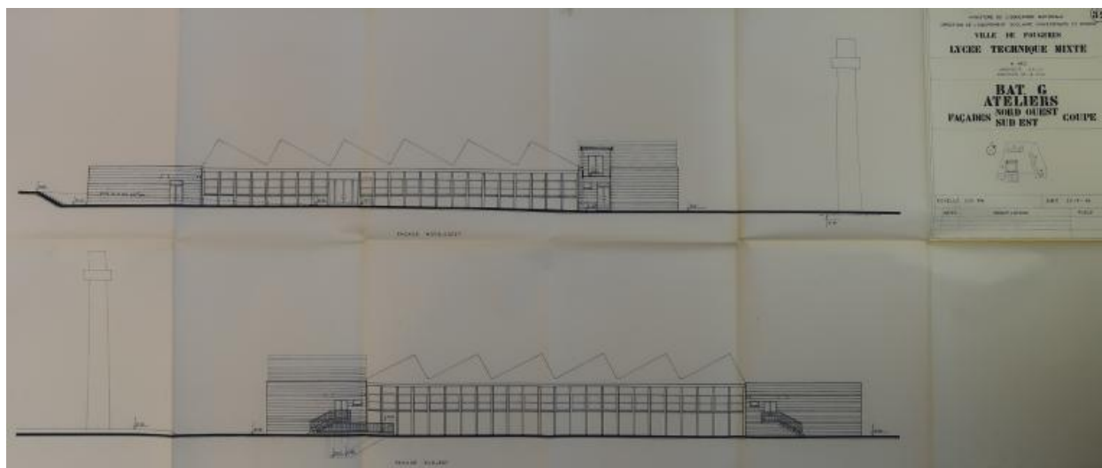
Bâtiment G, Ateliers. Façades nord-ouest - sud-est et Coupe. Albert Hec, architecte. 1964.
