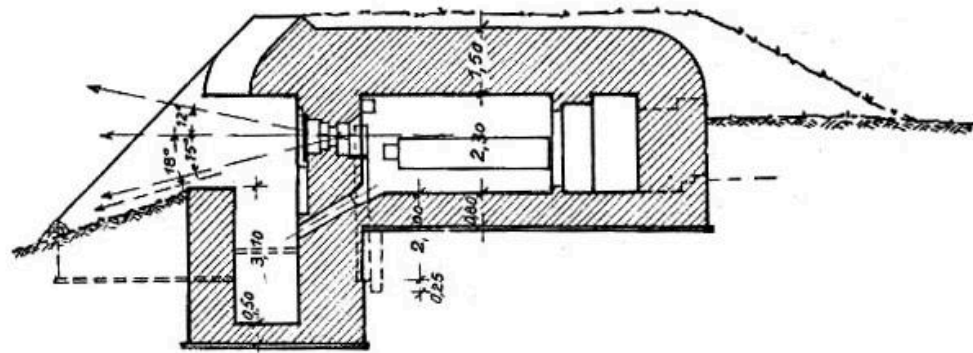
Schnitt A-B
