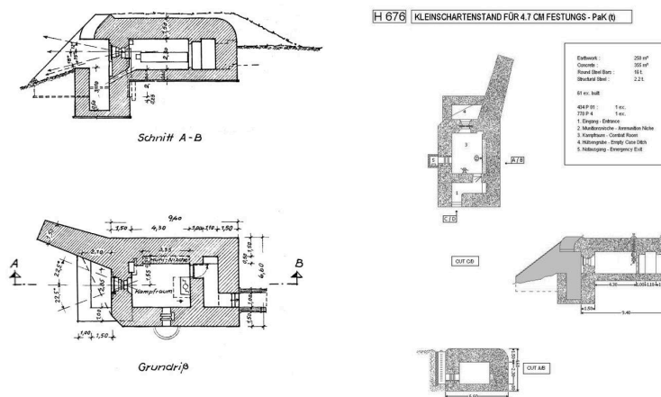
Plan-type d'un bunker de type 676 ( Kleinstschartenstand für 4,7 cm FestungsPaK ) Phot. Anonyme IVR53_20232905341NUCA
