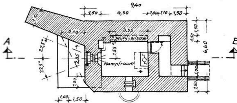
Grundriß
