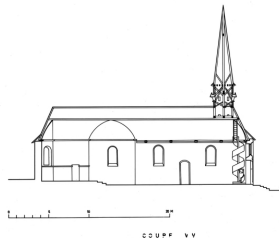
Coupe V-V. Repro. Norbert Lambart IVR53_19843501626P
