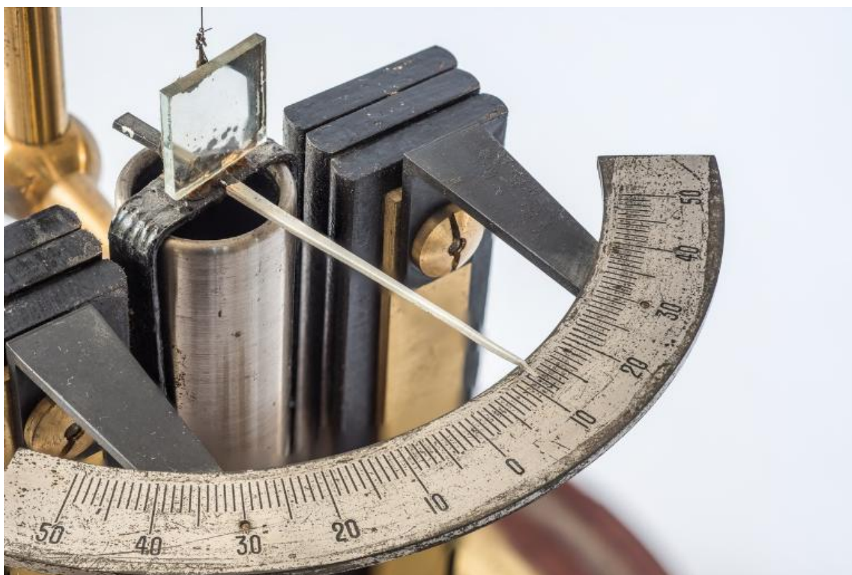
Détail du galvanomètre Deprez d'Arsonval
