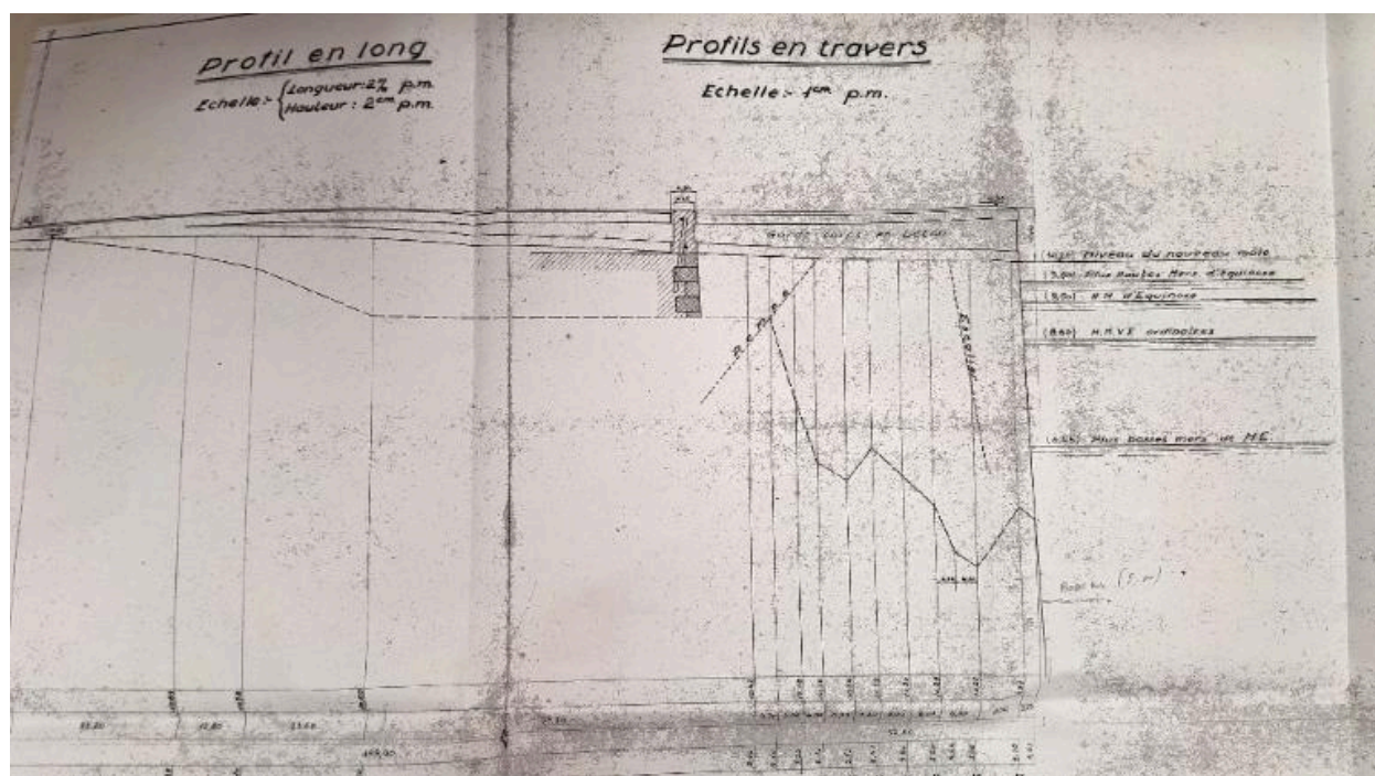
Coupe, profils de l'ouvrage de Pen ar Vil, juillet 1947
