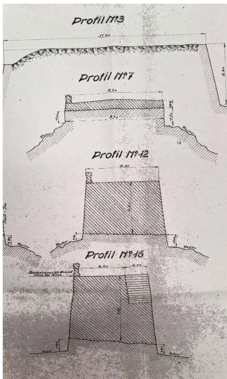
Profils de l'ouvrage de Pen ar Vil, juillet 1947
