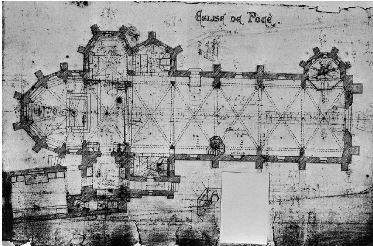
Plan au sol de l'église.
