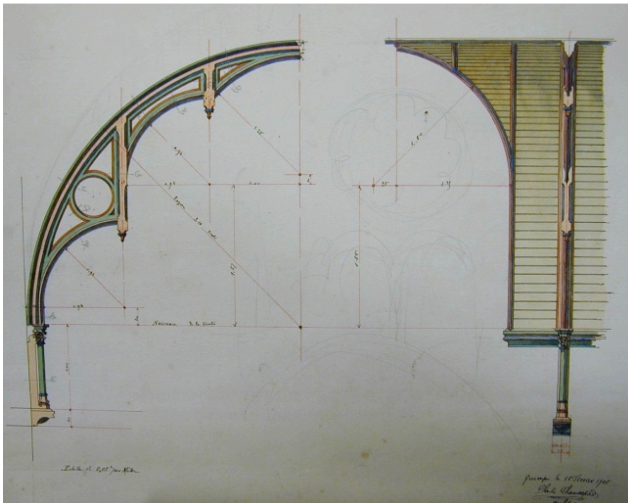
Rédené, église paroissiale Notre-Dame-de-Lorette : charpente. Dessin de Charles Chaussepied, 1905 (A.E. Quimper), reproduction de 2004
