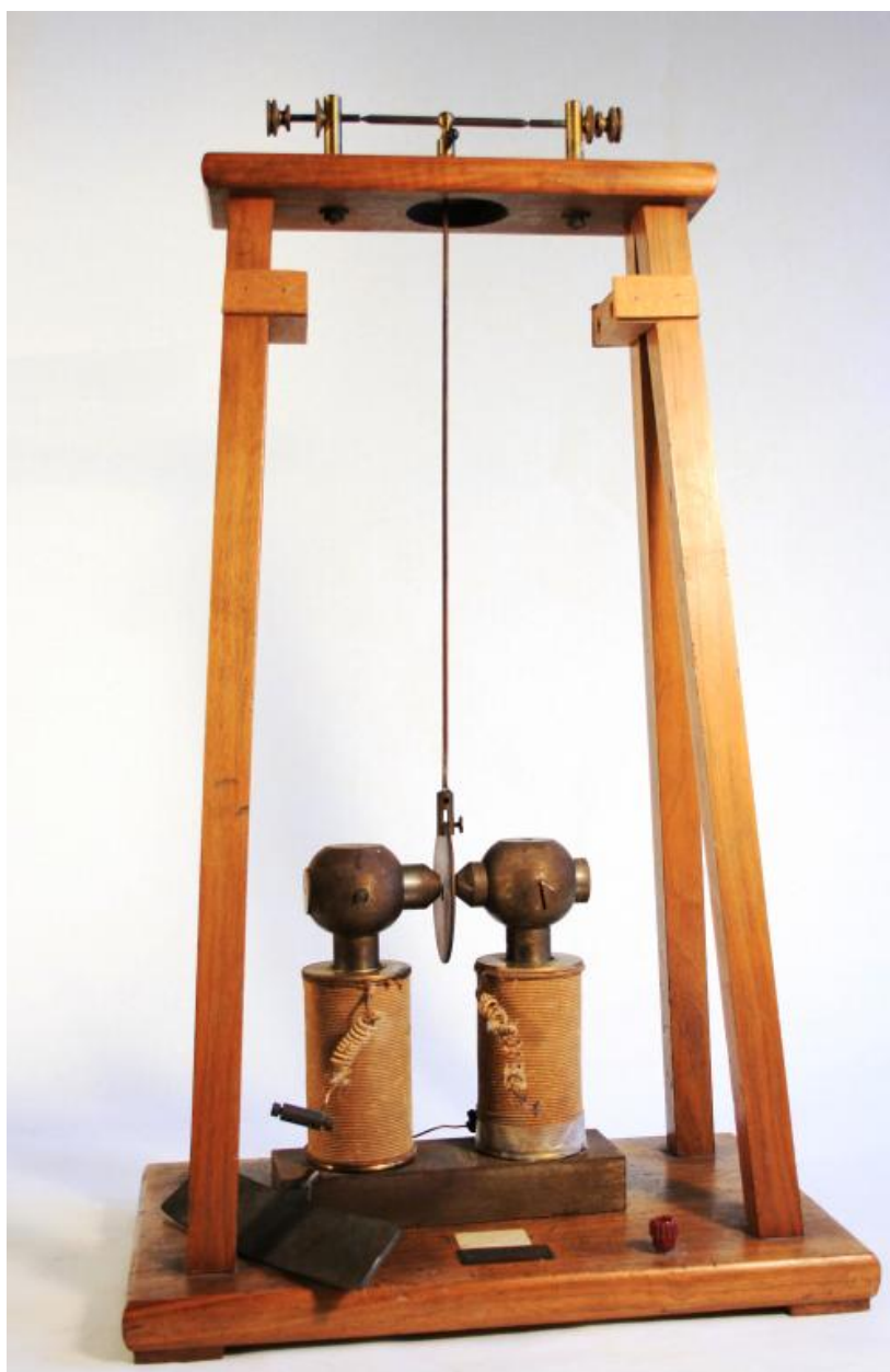
Electro-aimant Chassagny - Electricité dynamique (Radiguet & Massiot)
