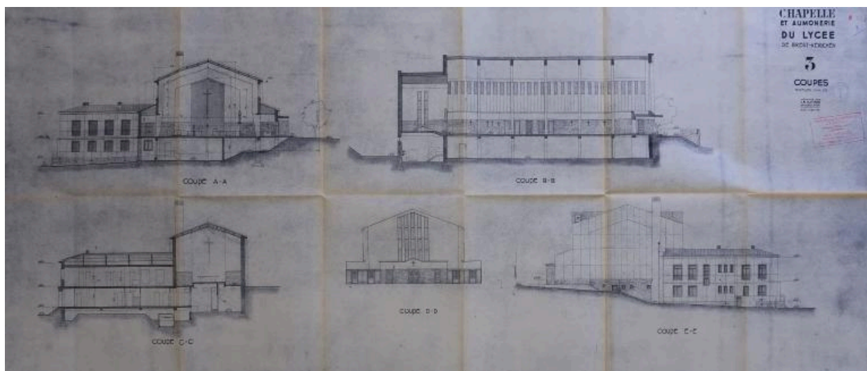
Chapelle et aumônerie du lycée. Coupes. Jean-Baptiste Mathon, architecte, 28.5.58.
