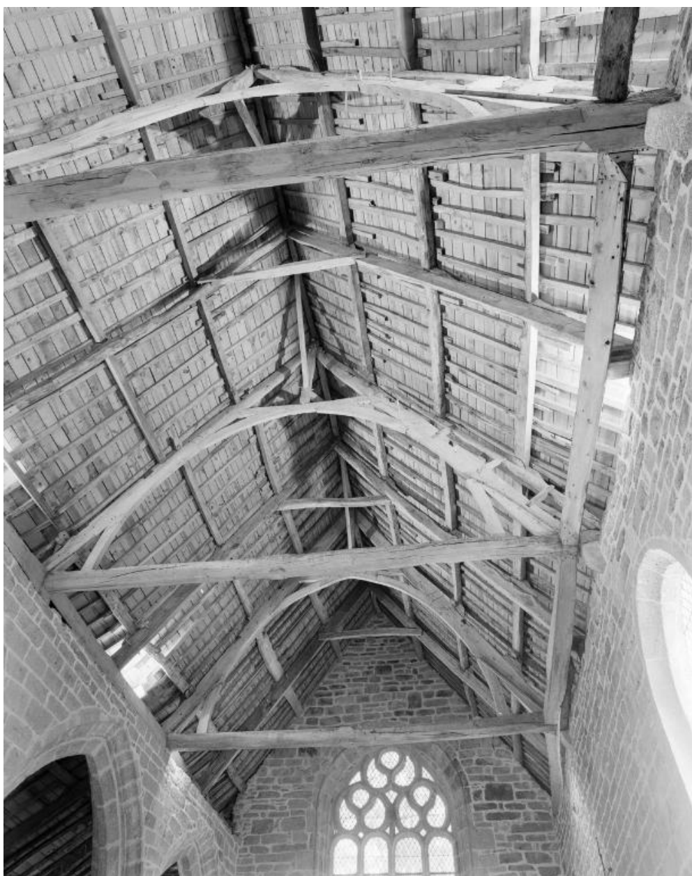
Vue générale de la charpente.
