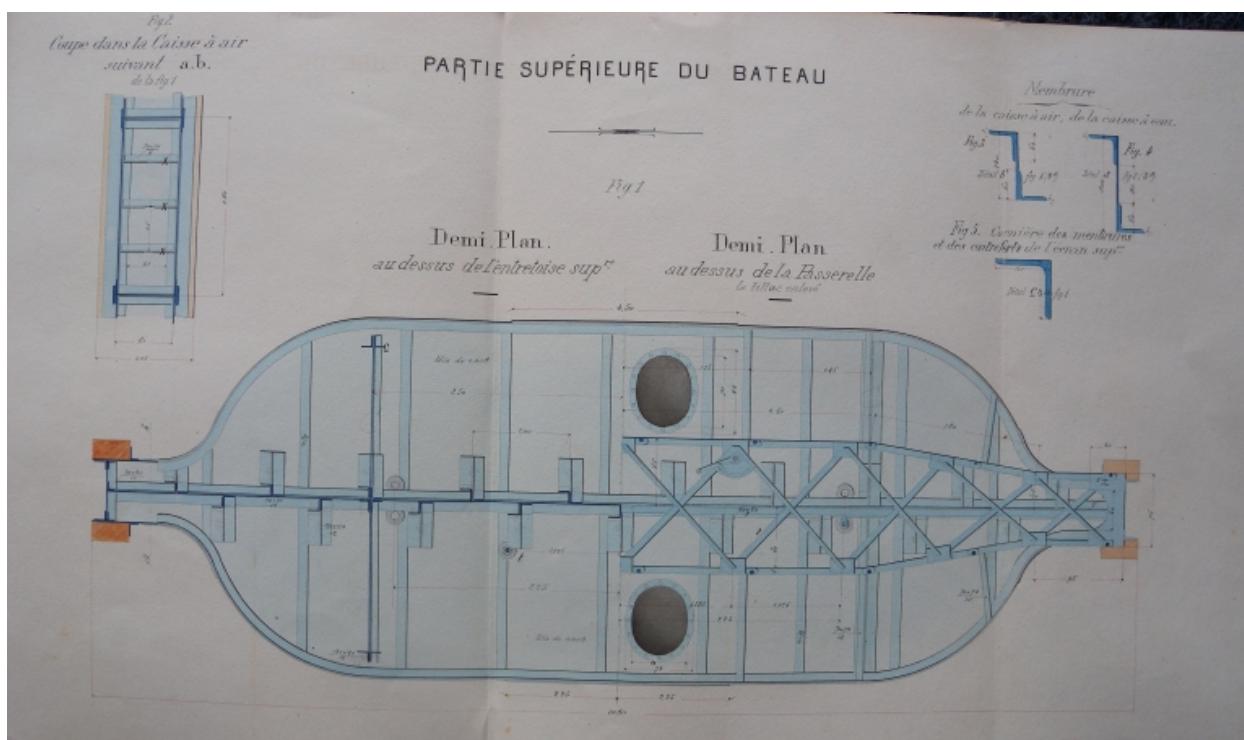
Plan : vue de la partie supérieure du bateau-porte, en projet, 1886 (AD 22)
