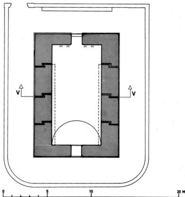
PLAN DU MAGASIN A POUVRE
