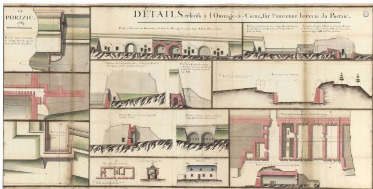
Détail relatif à l'ouvrage à corne sur l'ancienne batterie du Portzic (plans, coupes et élévations), 1784 (Collection : Archives départementales du Finistère)
