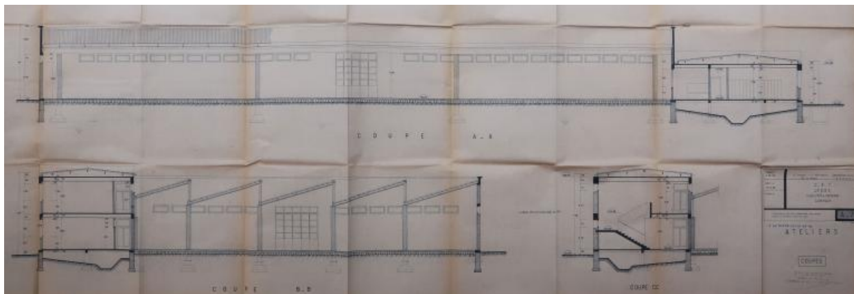
Ateliers : coupes. Hervé Péron et Alexandre Weisbein, architectes, 1964.
