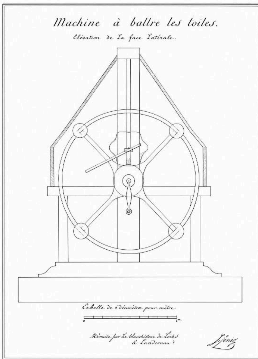
Machine à battre les toiles. Elévation de la face latérale. Dessin généré par l'IA, d'après un dessin original de Joseph-Guillaume Sénez (Lin et chanvre en Bretagne)
