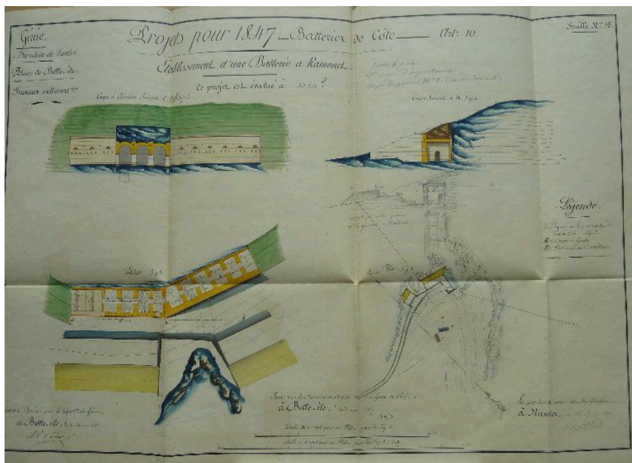
1 VH 292. Place de Belle-Ile, feuille n° 15 des projets extraordinaires pour 1847, établissement d'une batterie à Ramonet, 14 janvier 1847.
