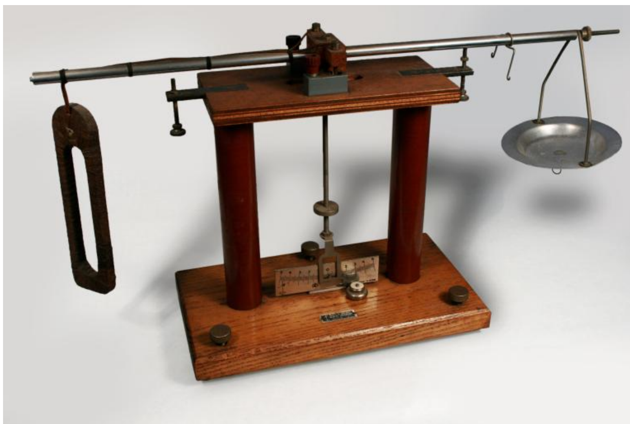
Maquette de la balance de Cotton - Electricité dynamique (Matériel de laboratoire Lefebvre)
