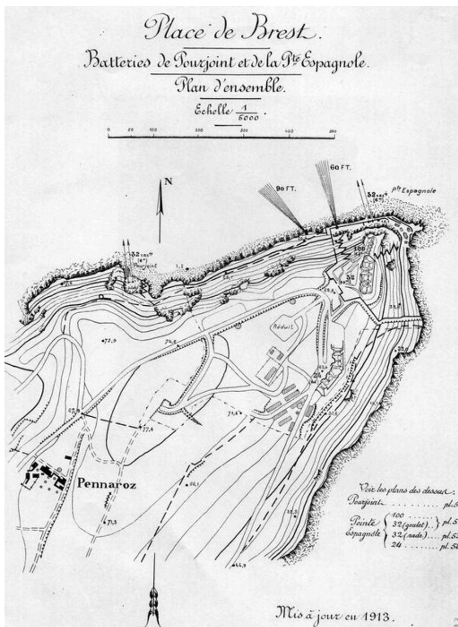
Plan de situation des batteries de Pourjoint et de la pointe des Espagnols, Atlas des batteries de côte : côte de Brest, 1913, Vincennes
