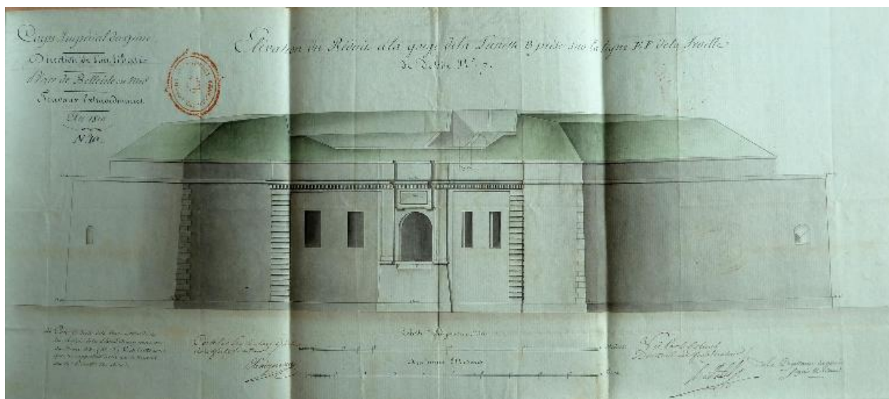
1 VH 286. Place de Belle-isle-en-mer, feuille n° 10 des projets pour 1810, élévation du réduit à la gorge de la lunette B.
