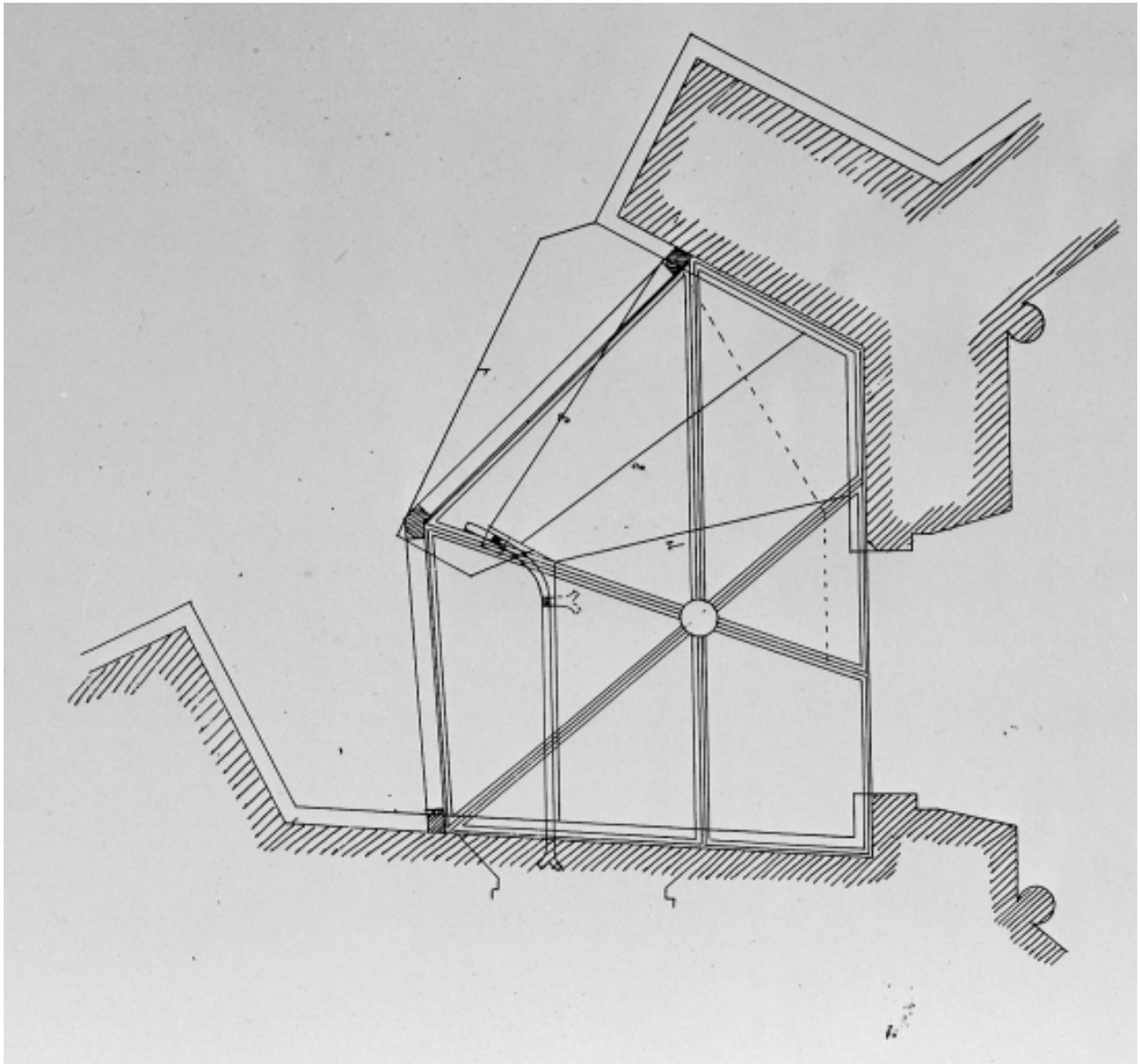
Plan du dais d'architecture au dessus d'une porte.
