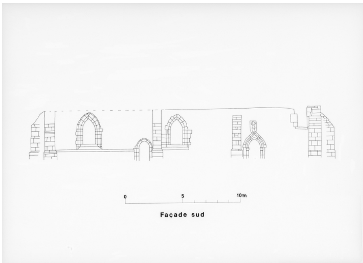
Elévation sud.
