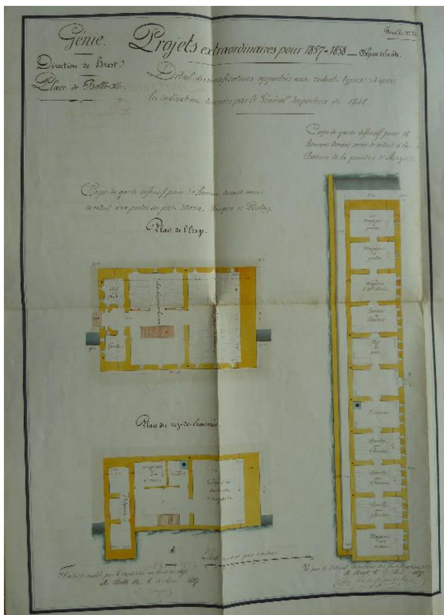
1 VH 294. Place de Belle-Ile, feuille n° 23 des projets extraordinaires pour 1857-1858, détail des modifications apportées aux réduits types, 18 mars 1857.
