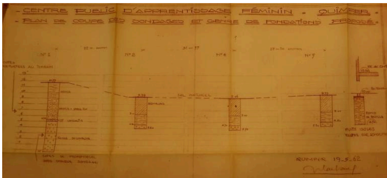
Plan de coupe des fondations et genre de fondations proposées. Centre public d'apprentissage féminin. Quimper. Jacques Lachaud, architecte, 19/05/1962.
