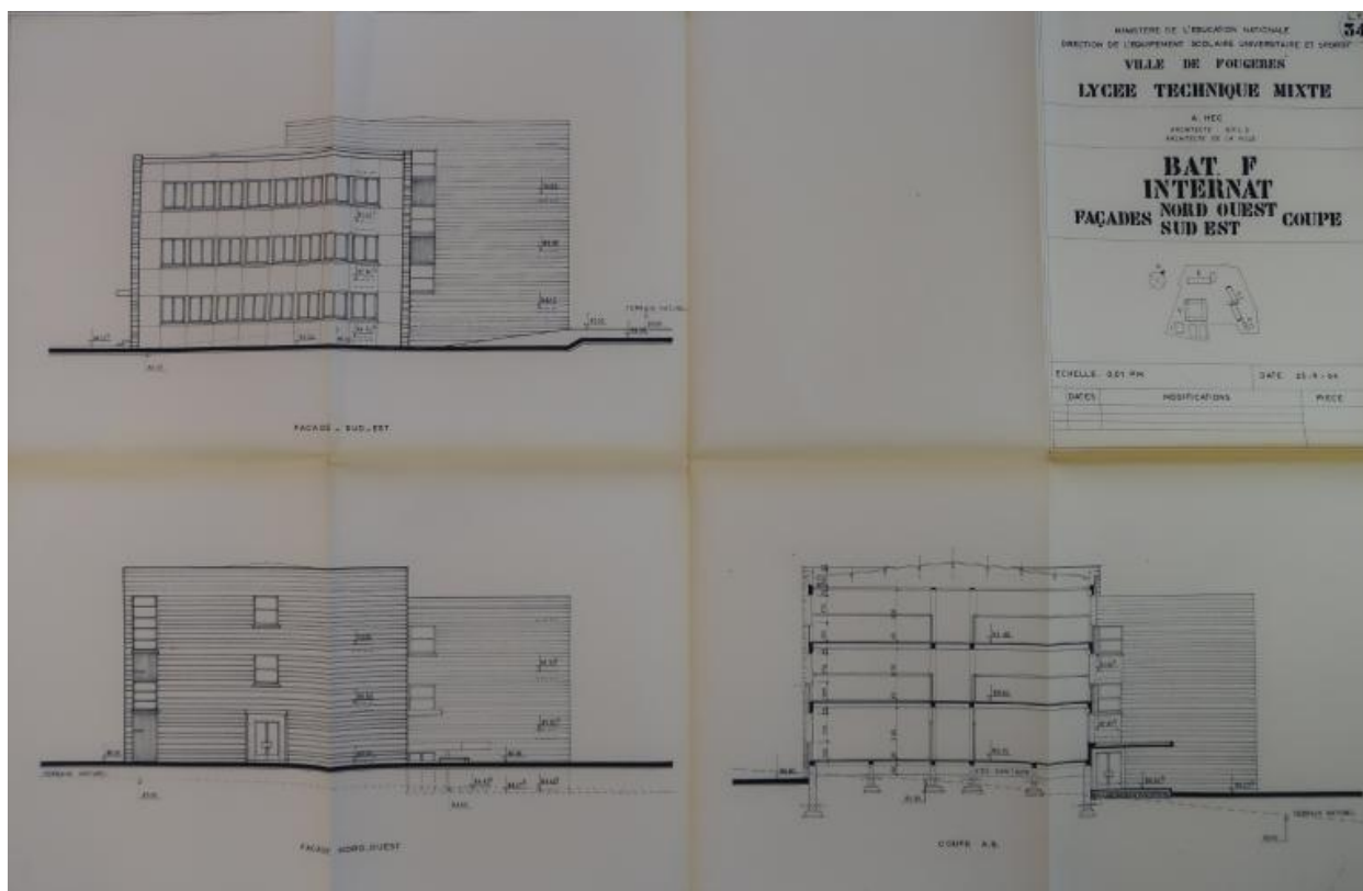
Bâtiment F, Internat. Façades nord-ouest et sud-est et Coupe. Albert Hec, architecte. 1964.
