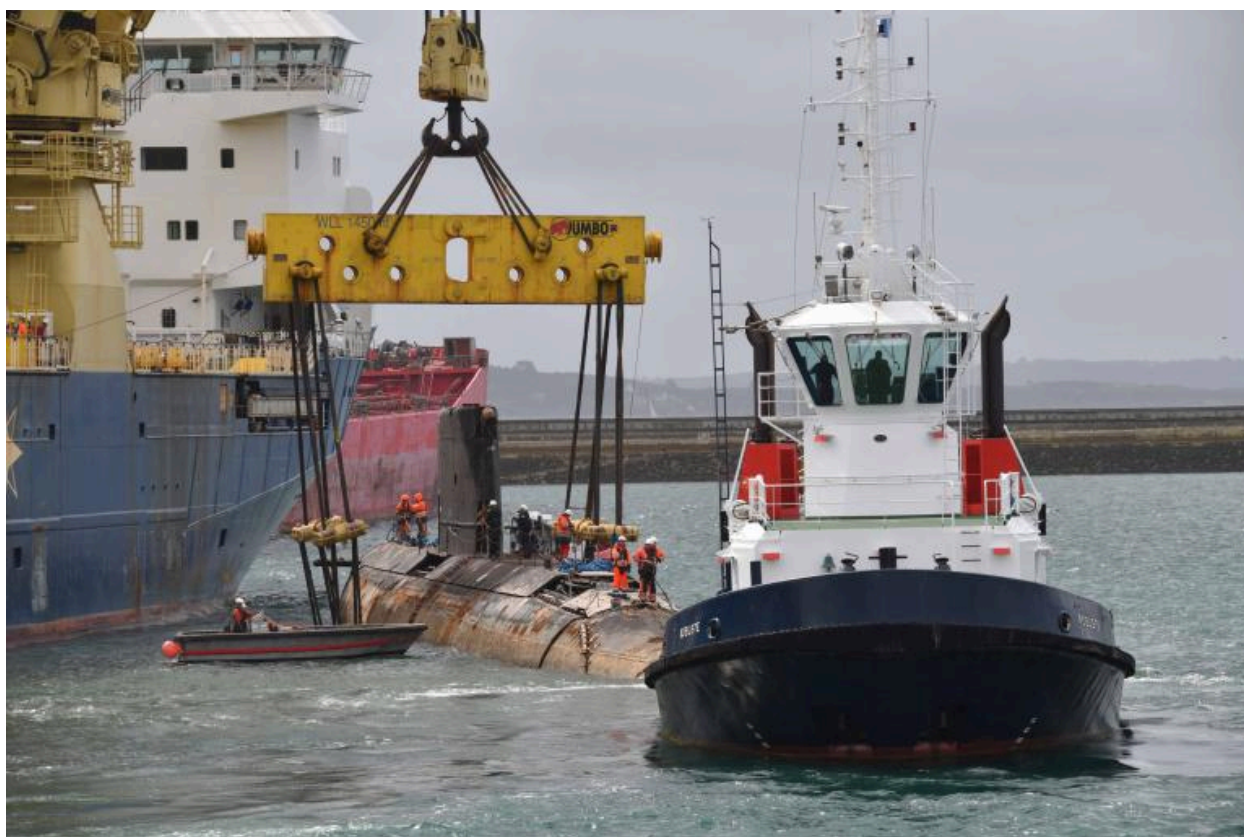
Déchargement de la coque de l'Agosta depuis le pont du Jumbo Kinetic au port de Brest, 5 août 2021
