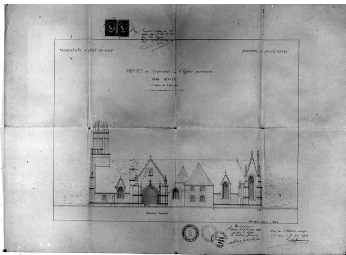
Projet de restauration de l'église, état actuel 1894 : plan, coupe et élévation de la façade ouest (reproduction)
