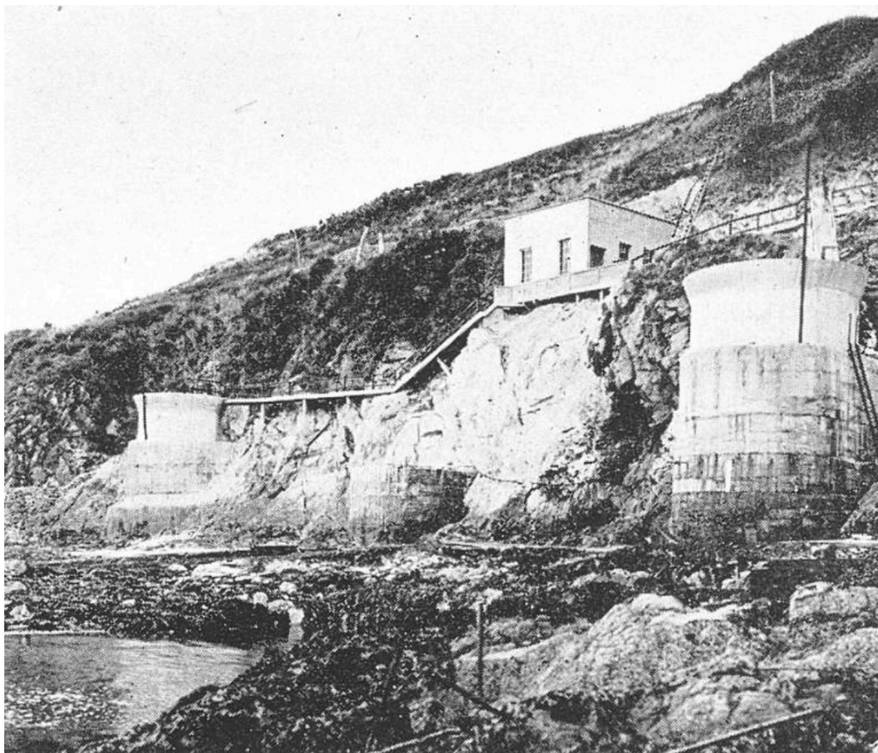
Vue de l'ouvrage de prise d'eau de mer depuis la grève, novembre 1953
