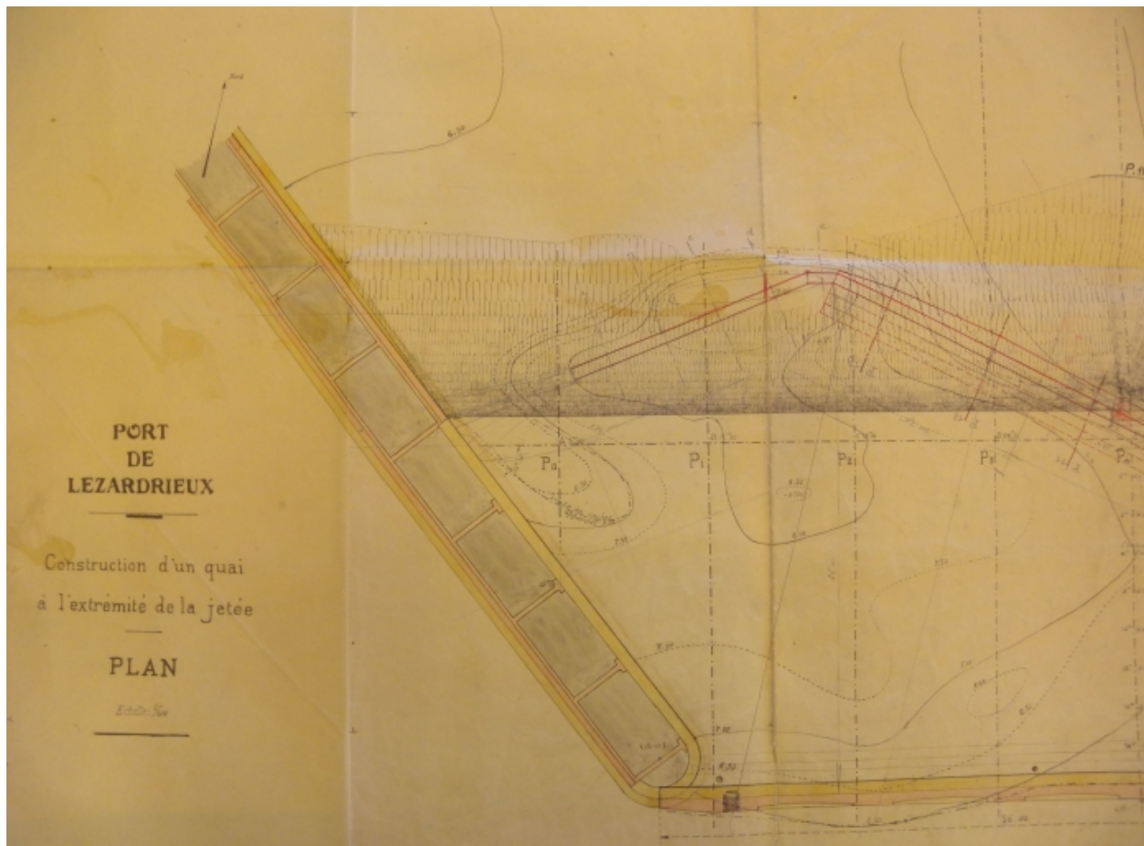
Plan : élévation du nouveau quai sur voûtes et de la jetée, 1927 (AD 22)
