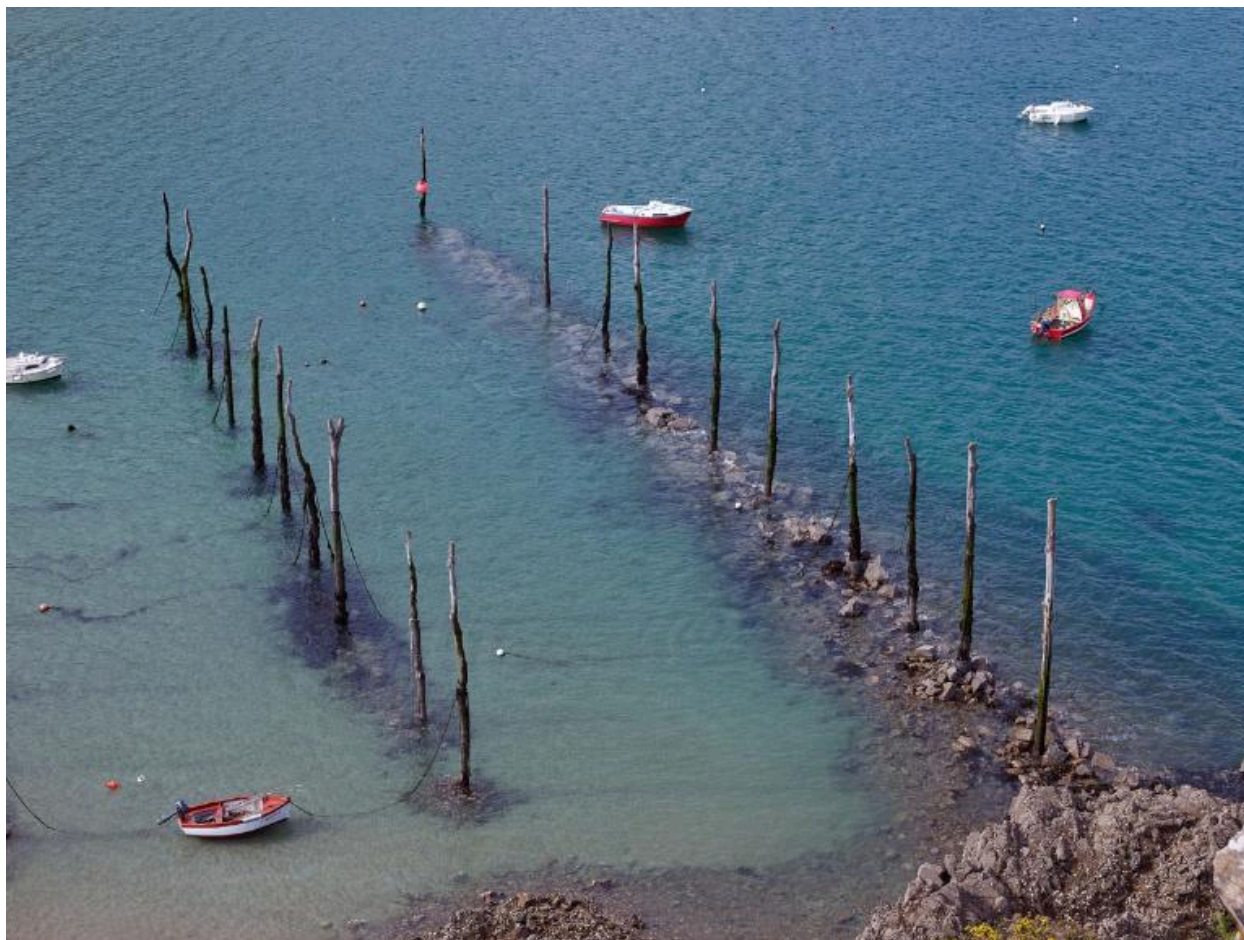
Alignement d'enrochement pour maintenir les pieux de mouillage et formant brise-houle
