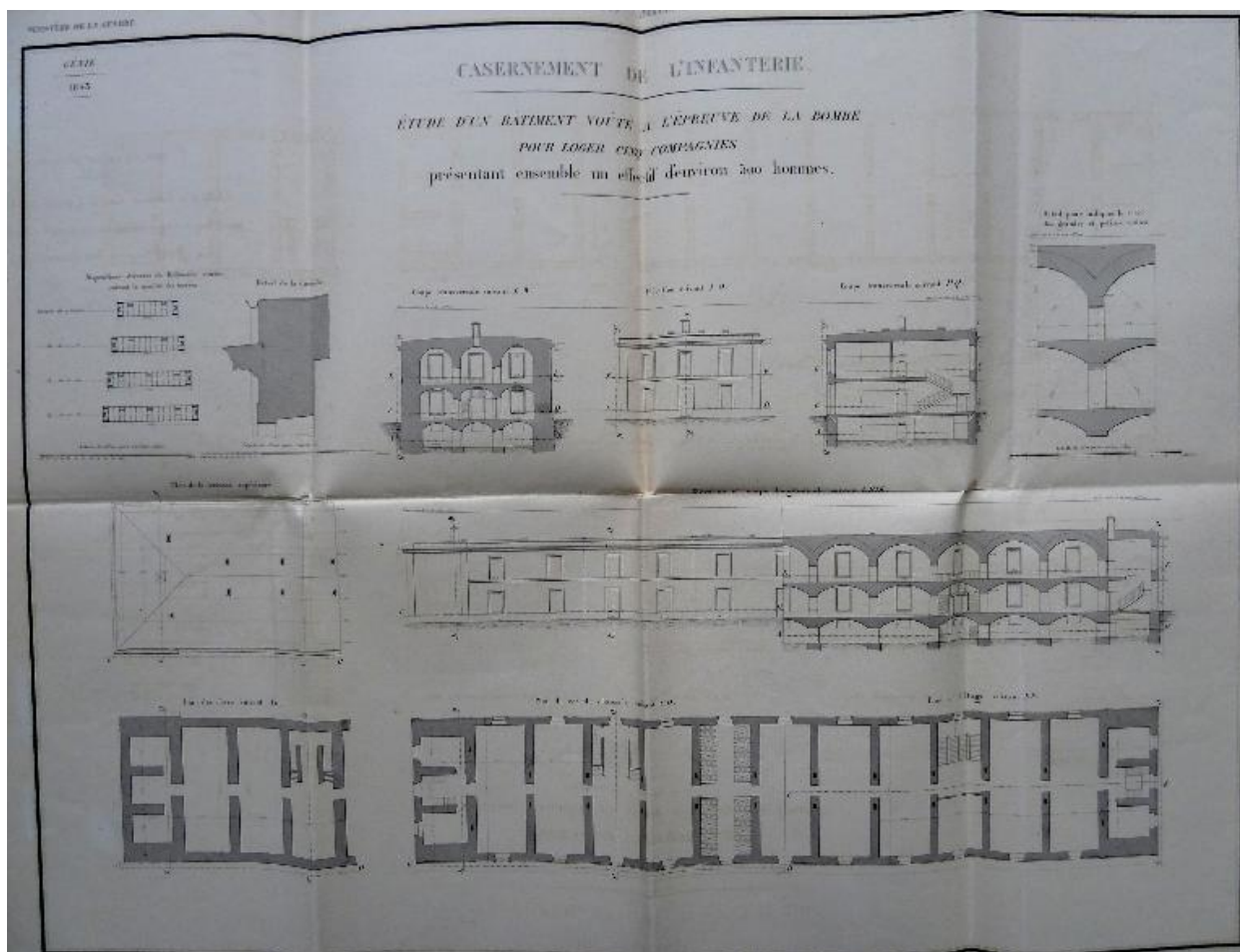
1 VK 139. Étude d'un bâtiment voûté à l'épreuve de la bombe pour loger cinq compagnies, 1843.
