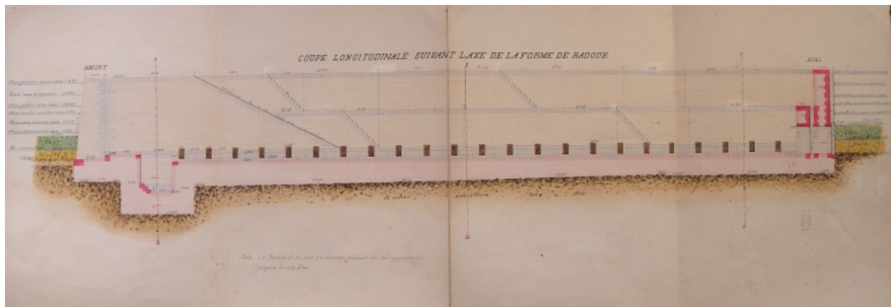
Plan : coupe longitudinale de la forme de radoub, 1883 (AD 22)
