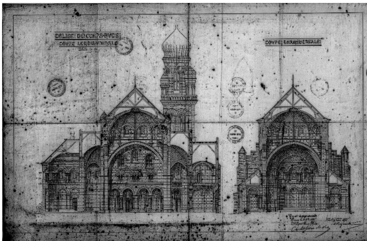
Coupes longitudinale et transversale
