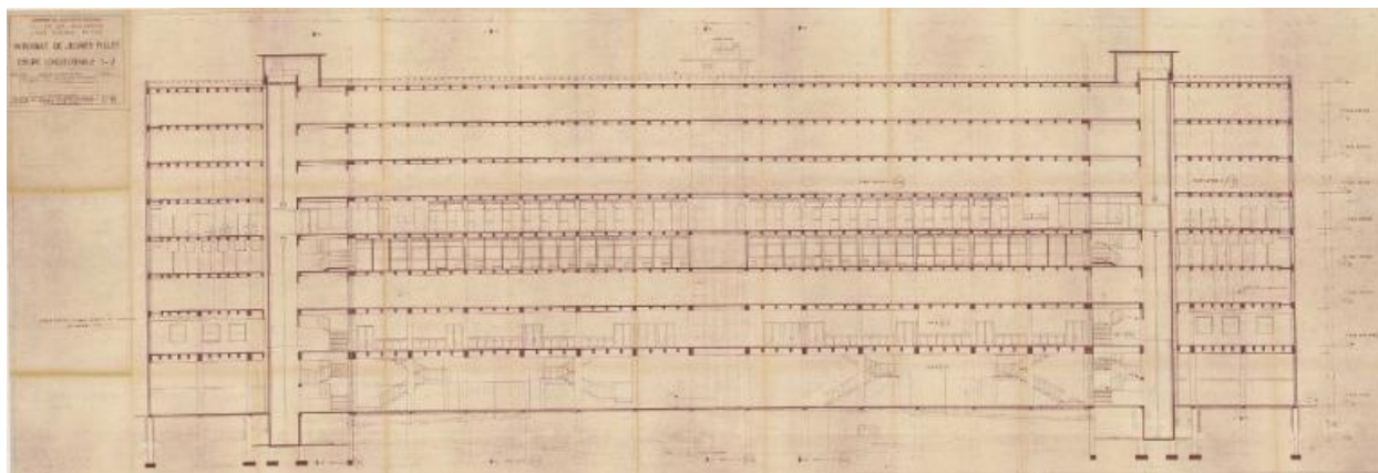
Internat de jeunes filles. Coupe longitudinale. Raymond Lopez, architecte, 1952.
