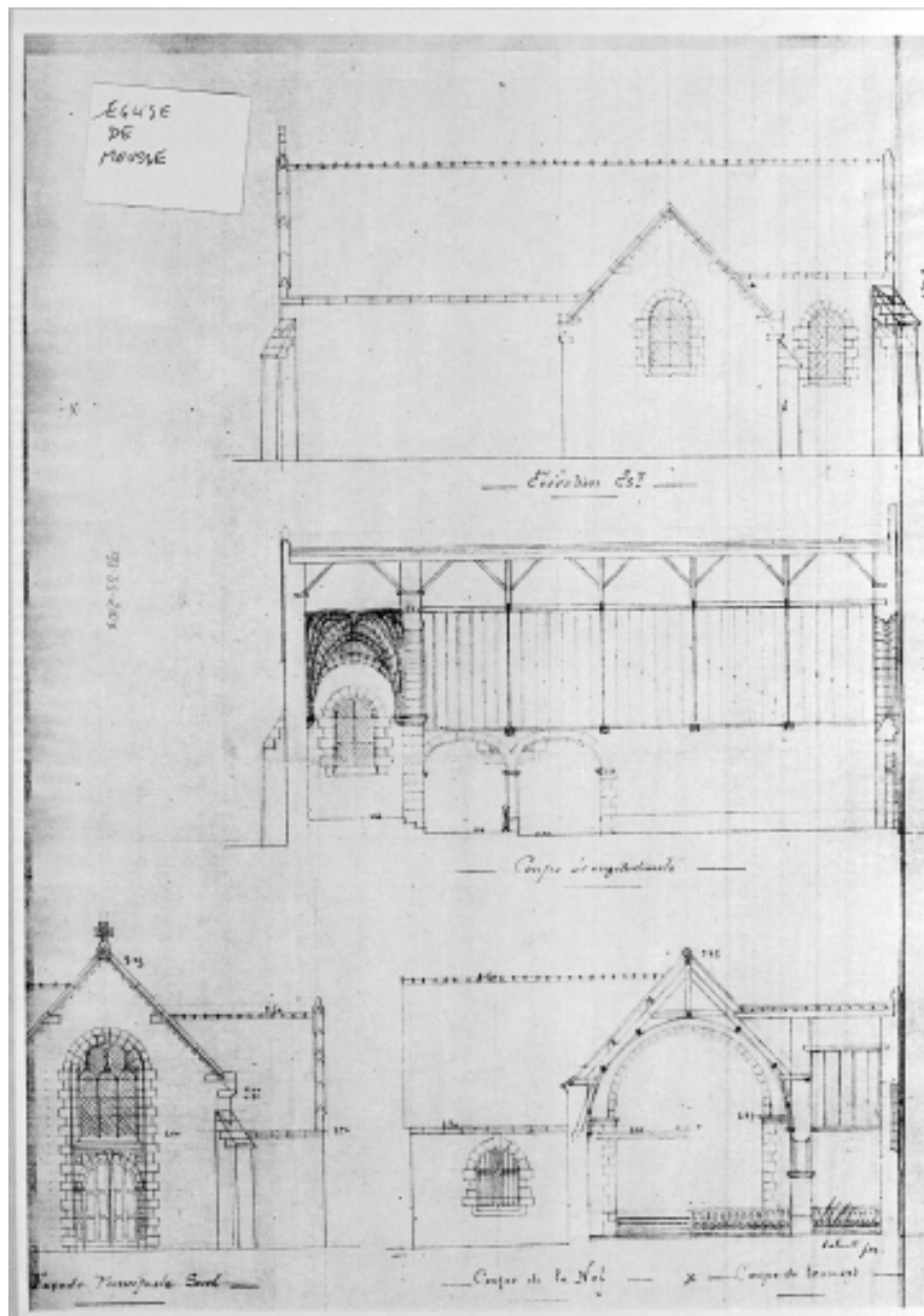
Coupe longitudinale
