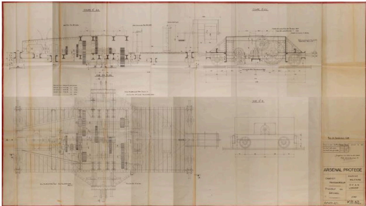
Plans et coupes du chariot transbordeur et tracteur électrique du berceau, plan KB n° 60, 27 novembre 1967 (Service Historique de la Défense de Lorient, Monographie de la base "Ingénieur Général Stoskopf")
