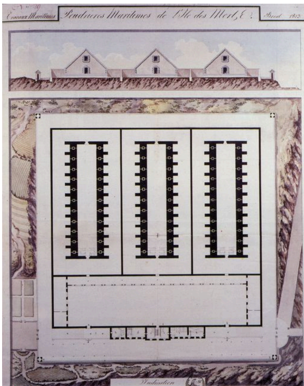
Plan et élévation des trois magasins à poudre dits "poudrières maritimes" de l'île des Morts, Travaux Maritimes, 1813
