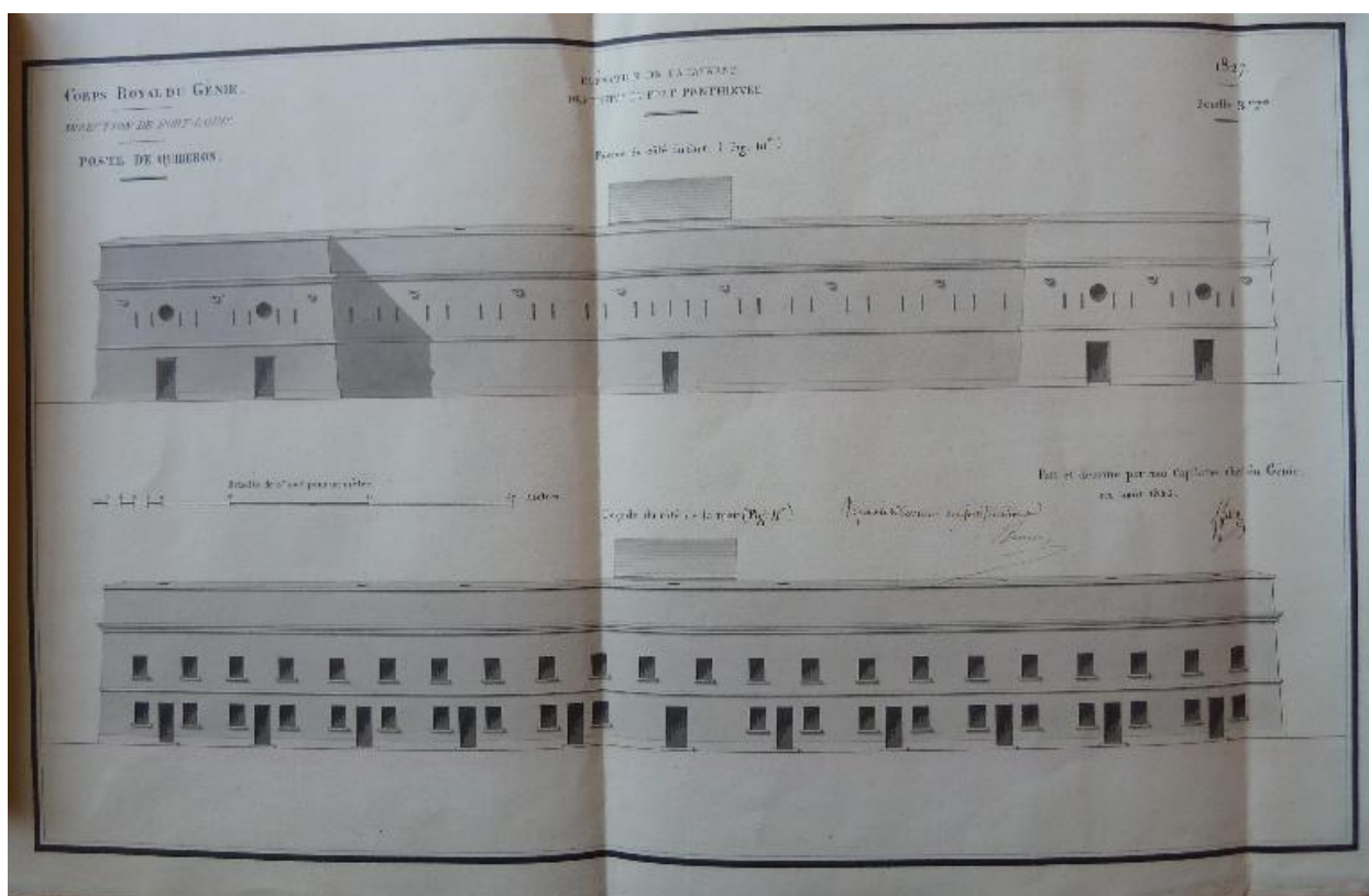
1 VH 1516. Direction du Génie de Port-Louis, Poste de Quiberon, feuille n° 3 des projets pour 1827, élévation de la caserne défensive du fort Penthièvre, août 1826.
